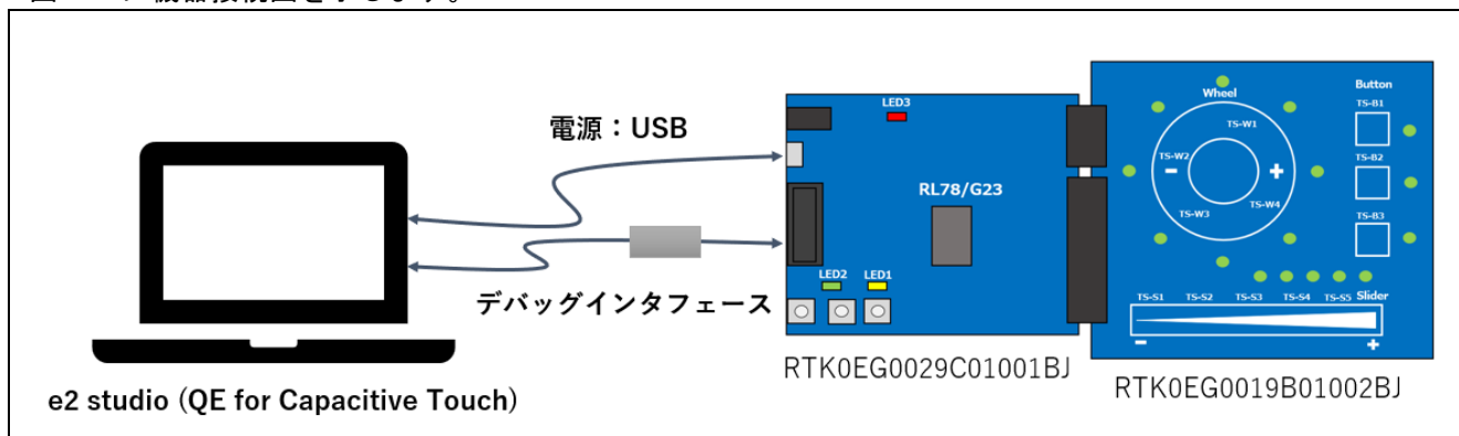
図 2.1 機器接続図
