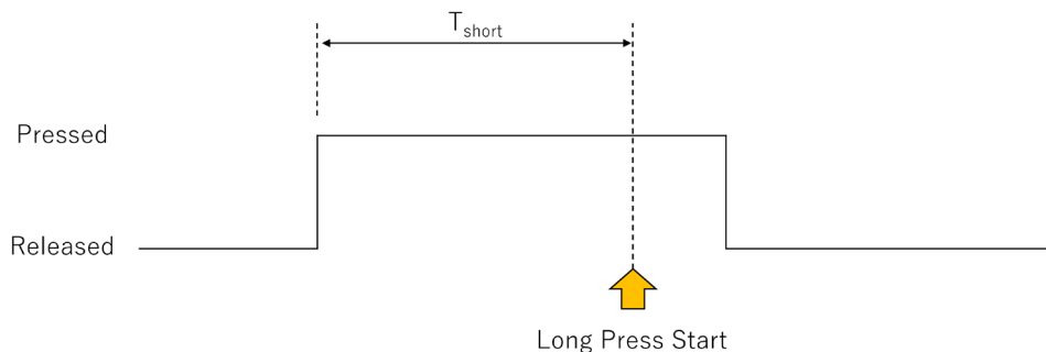
図 4-8 Long Press Repeat イベント発生条件
