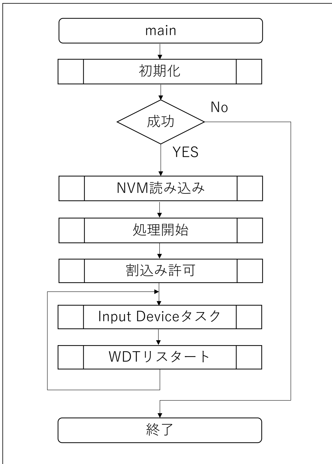
図 4-16 メインフロー図
