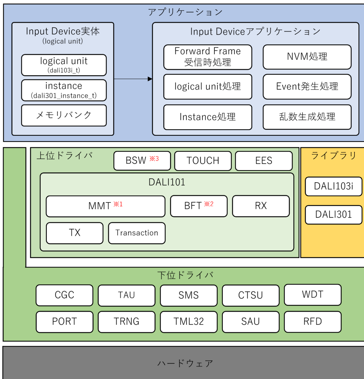
図 4-10 機能ブロック図
