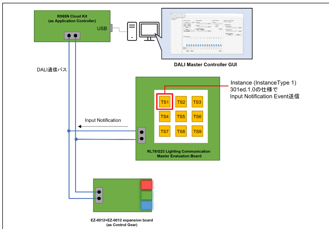
図 4-9 システム構成例(RX65N Cloud kit + DALI-2 オプションボード使用)
