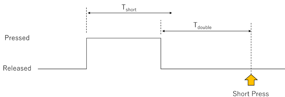
図 4-6 Double Press イベント発生条件
