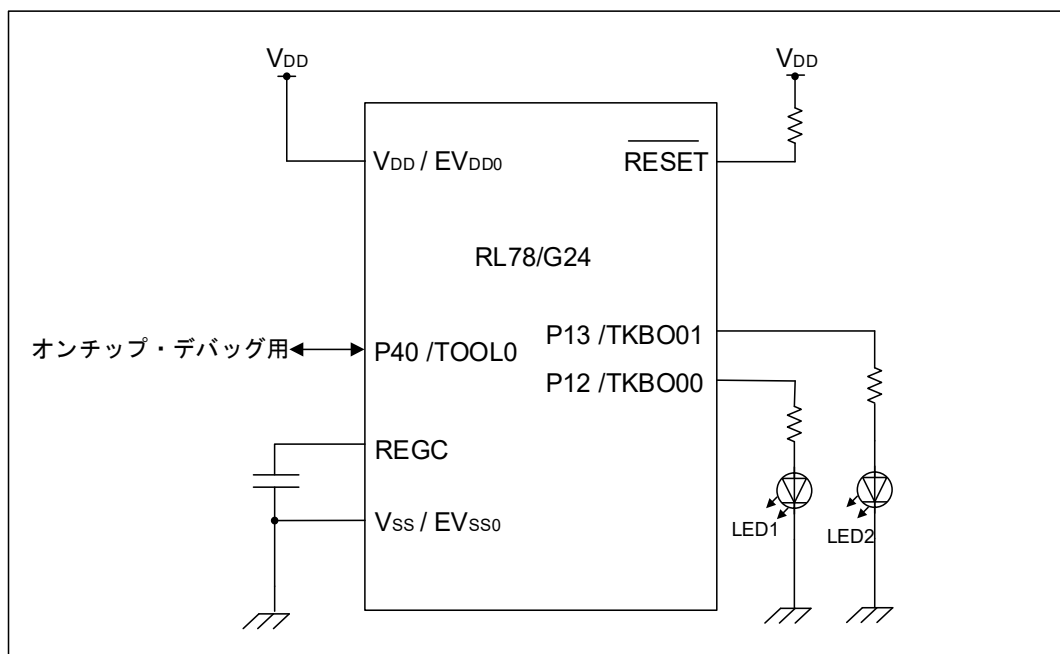
図 3-2 ハードウェア構成例
