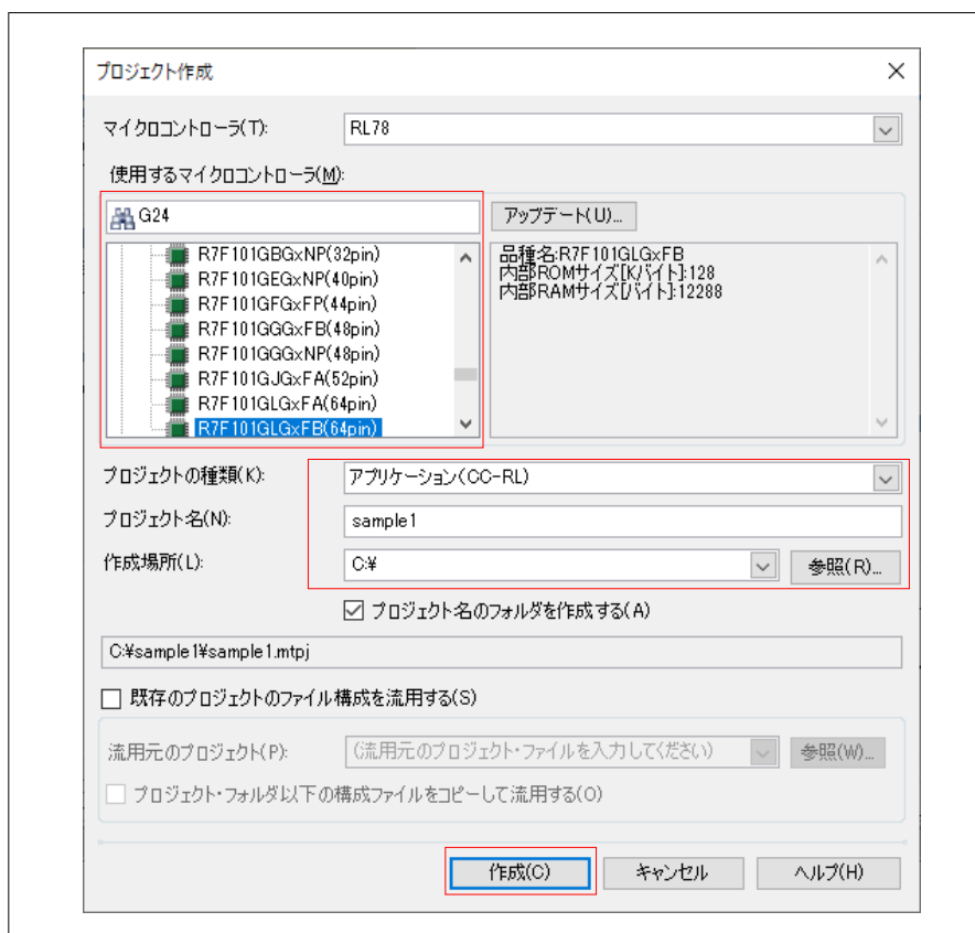
図 2-2 プロジェクト作成ダイアログ
