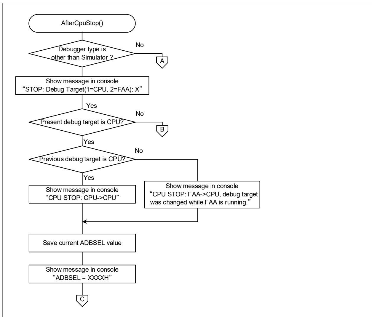
図 3-18 AfterCpuStop 処理 (1/2)
