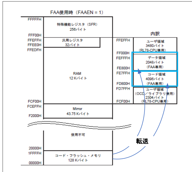
図 1-5 FAA のプログラムとデータの転送
