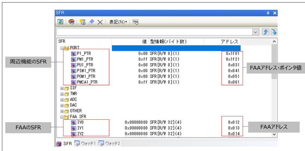
図 2-43 SFR パネル
