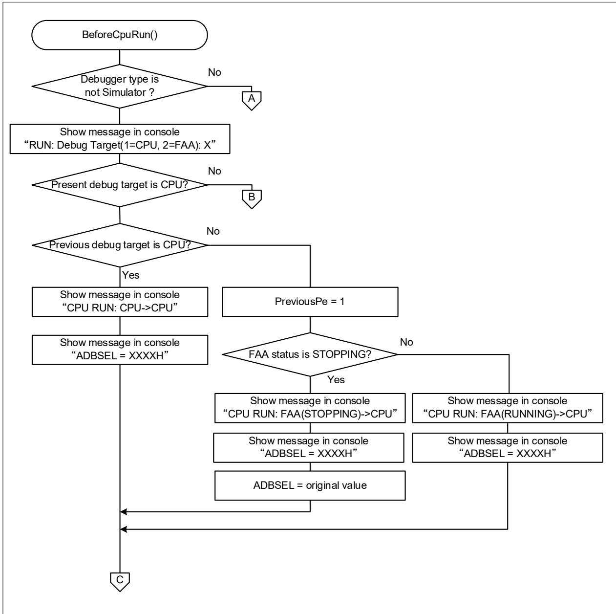
図 3-16 BeforeCpuRun 処理 (1/2)
