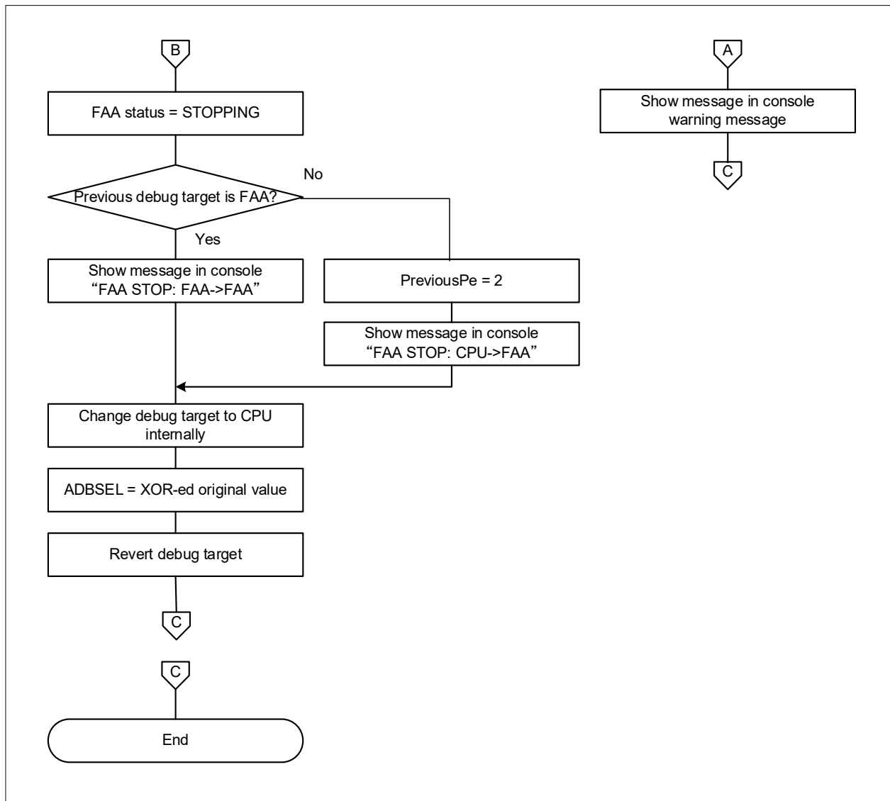
図 3-19 AfterCpuStop 処理 (2/2)
