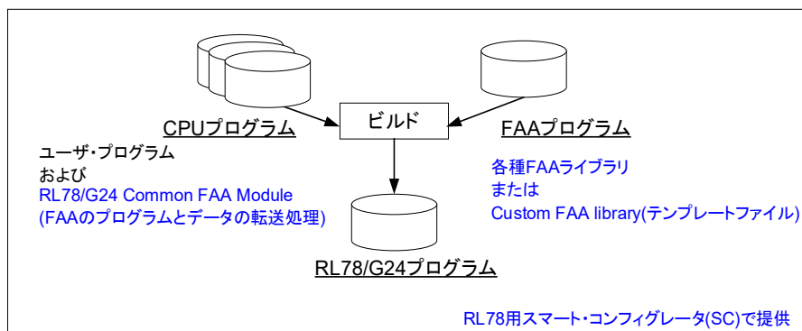
図 1-4 RL78 用スマート・コンフィグレータで提供する FAA 関連のファイル
