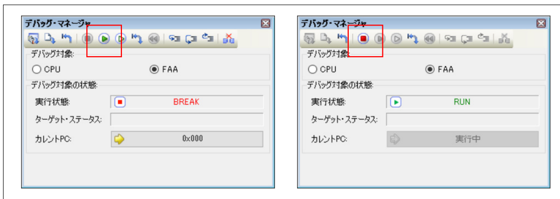
図 2-37 デバッグ・マネージャ
