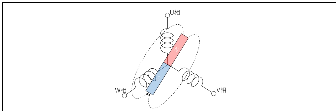
図 3-14 回転子位置と各相の関係
