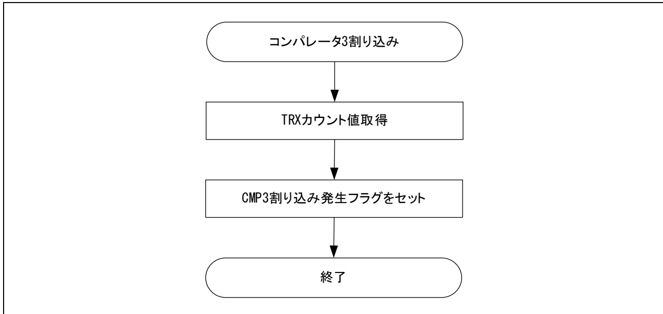
図 3-32 コンパレータ 3 割り込み処理フローチャート
