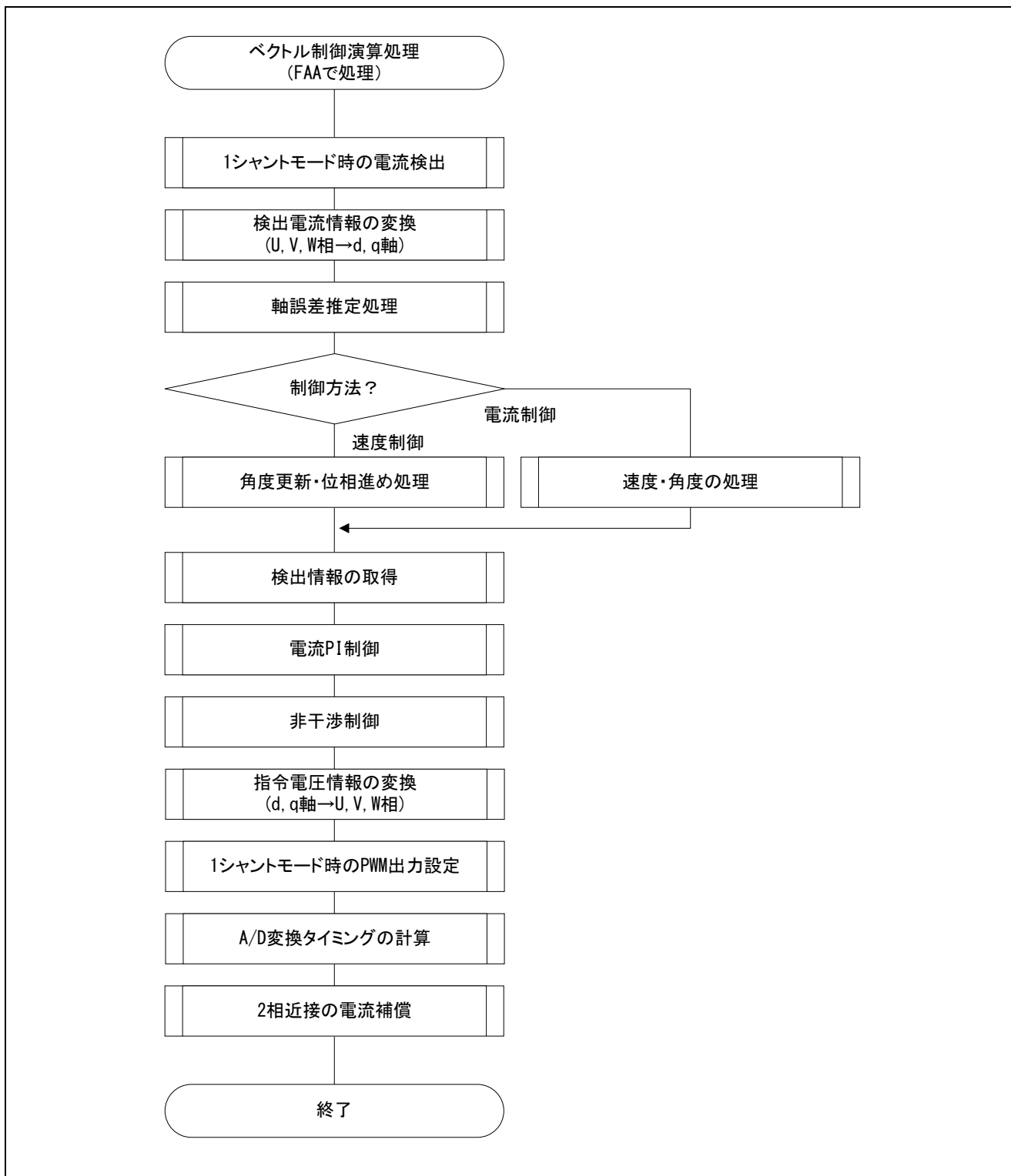
図 3-28 ベクトル制御演算処理 (1 シャントモード時) フローチャート
