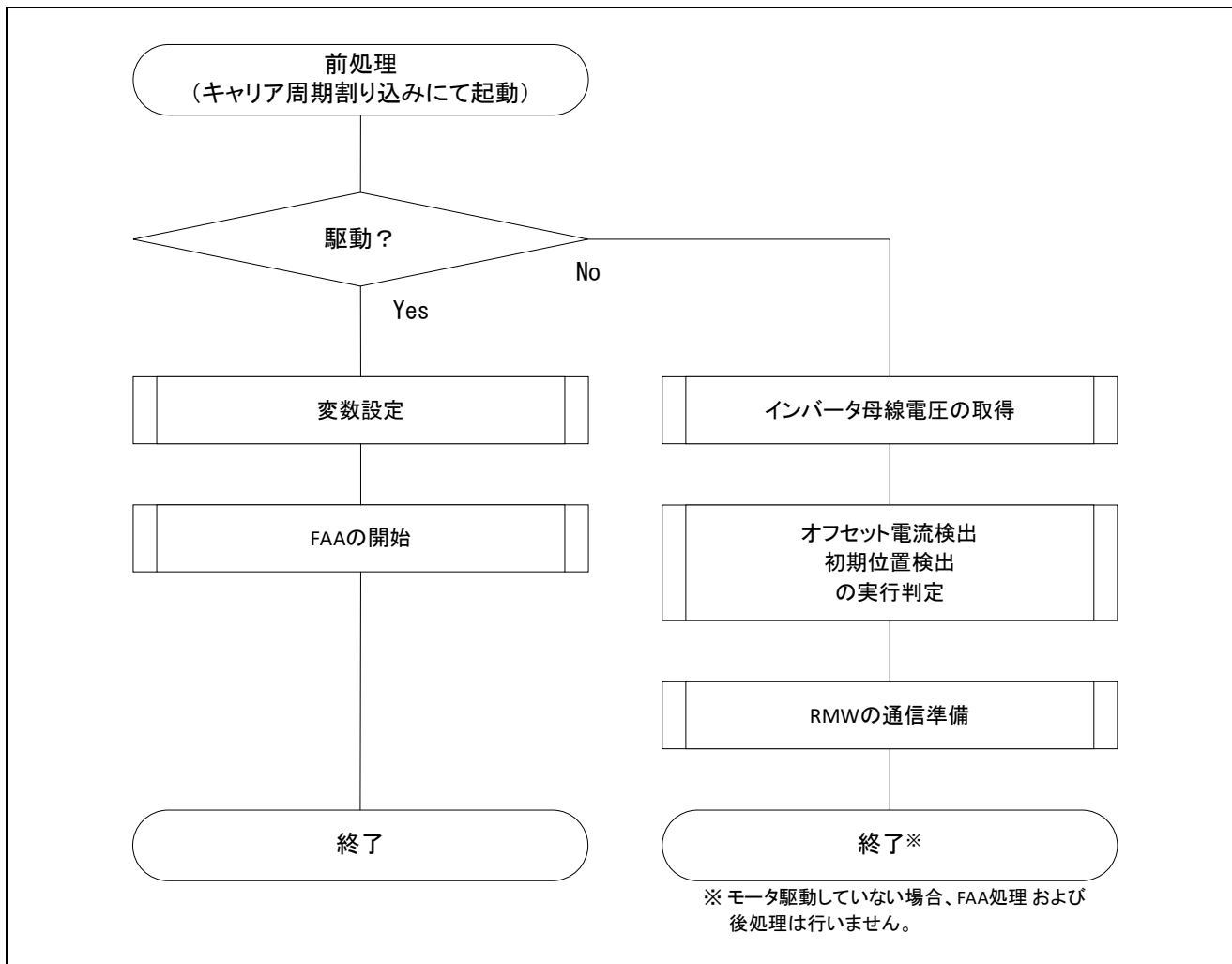
図 3-27 前処理フローチャート
