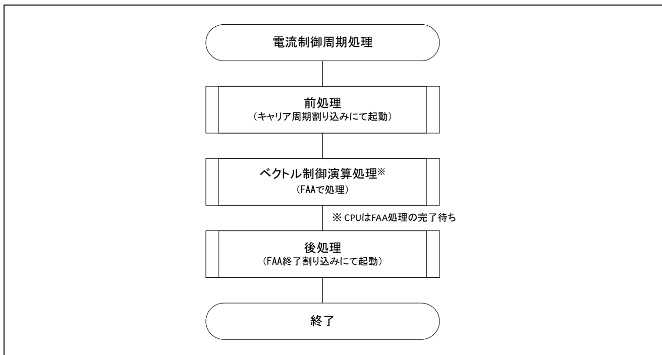
図 3-26 電流制御周期処理フローチャート
