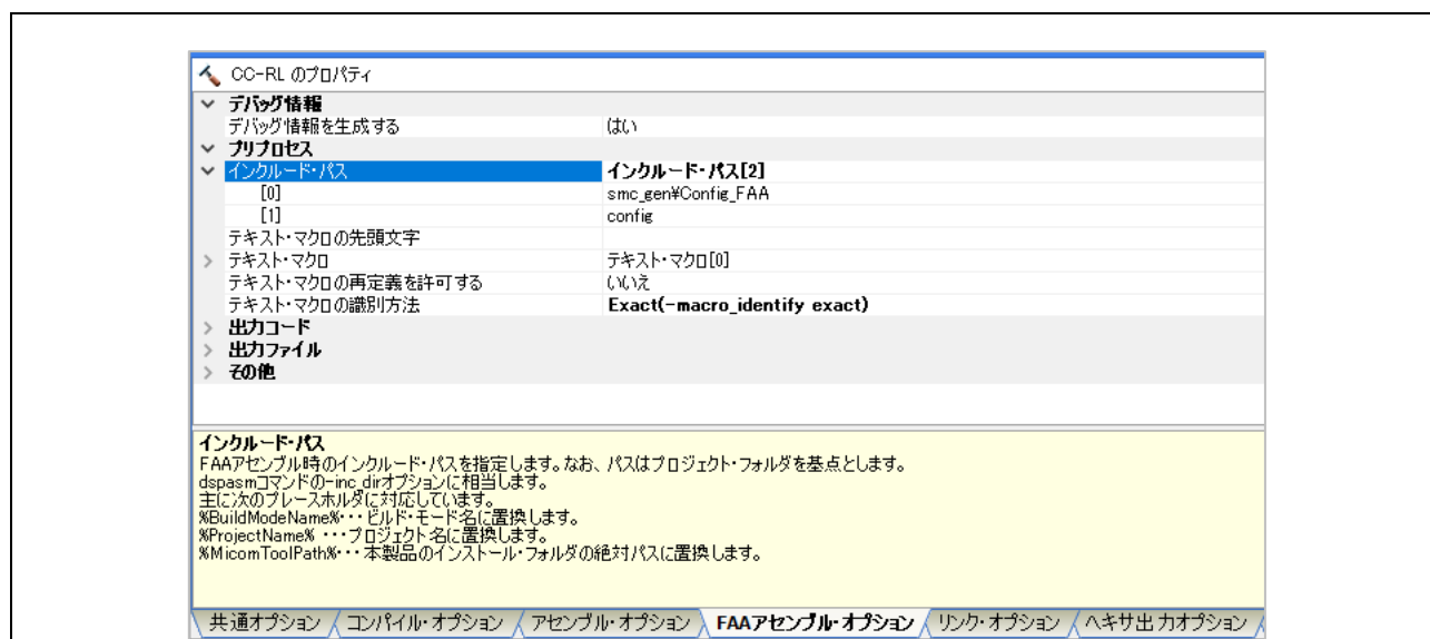
図 5-1 CS+でのインクルード・パス設定
