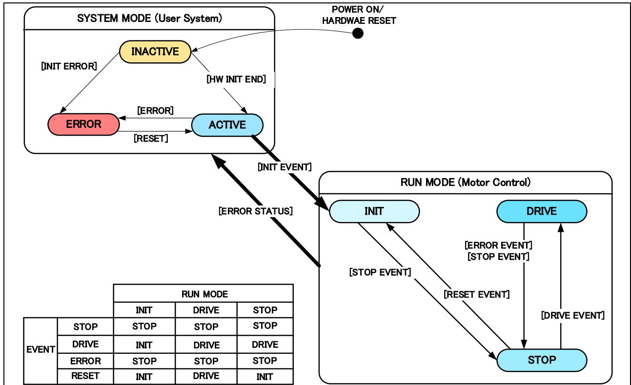
図 3-4 状態遷移図
