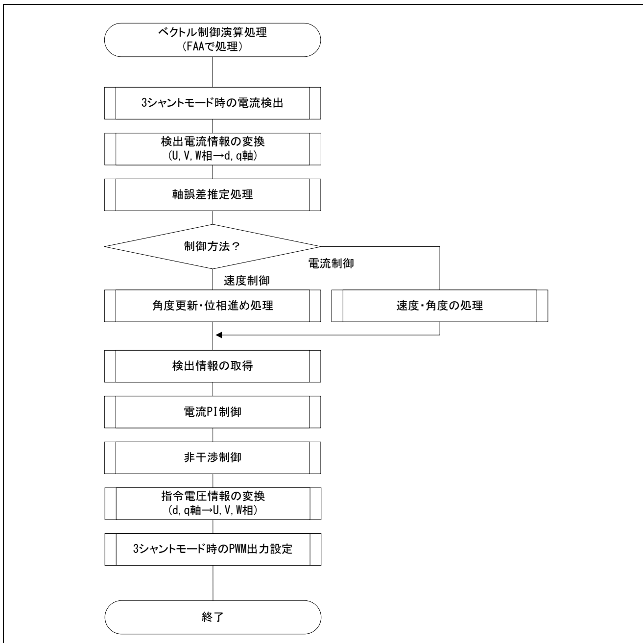
図 3-29 ベクトル制御演算処理 (3 シャントモード時) フローチャート
