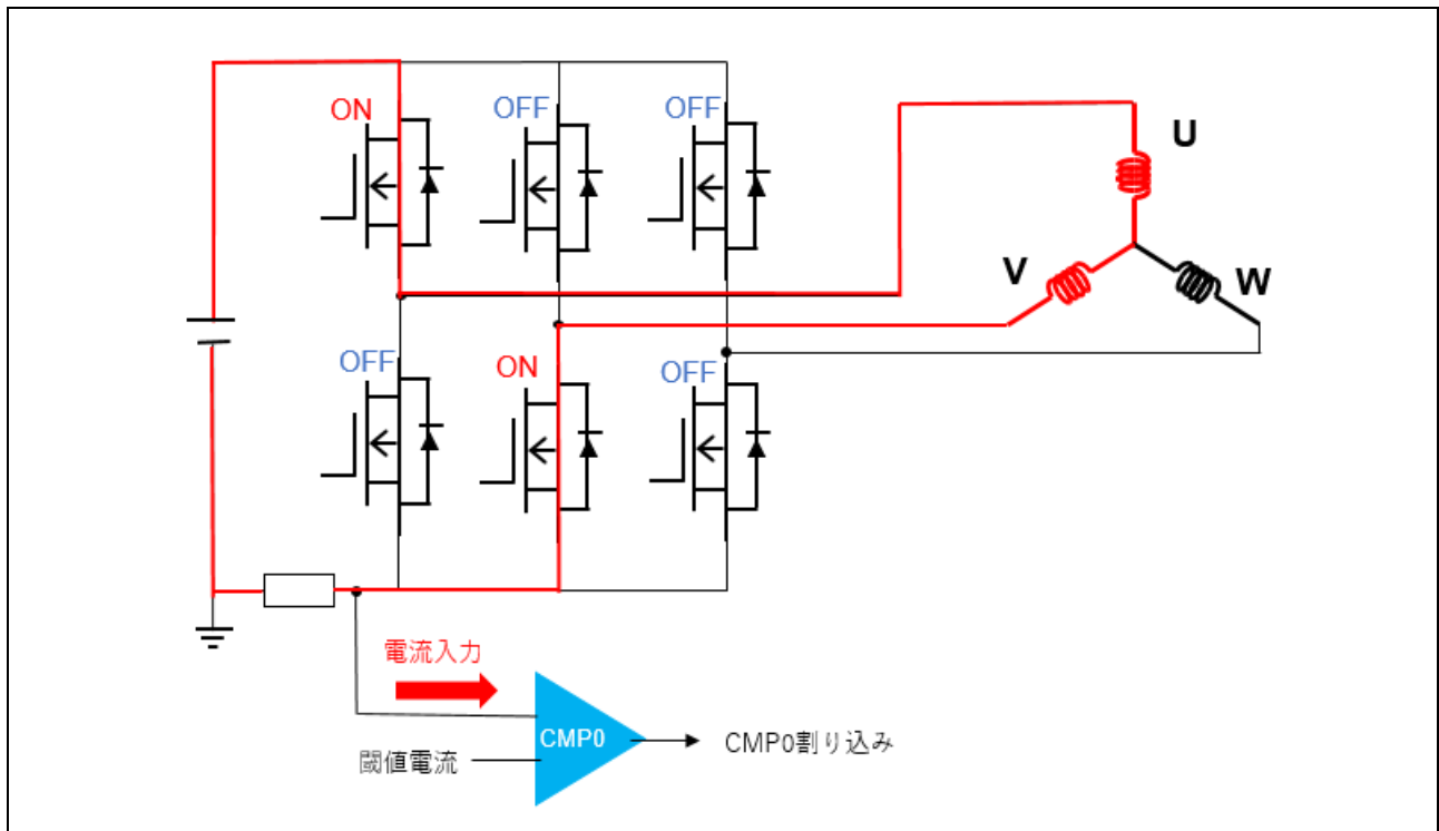
図 3-15 角度検出模式図
