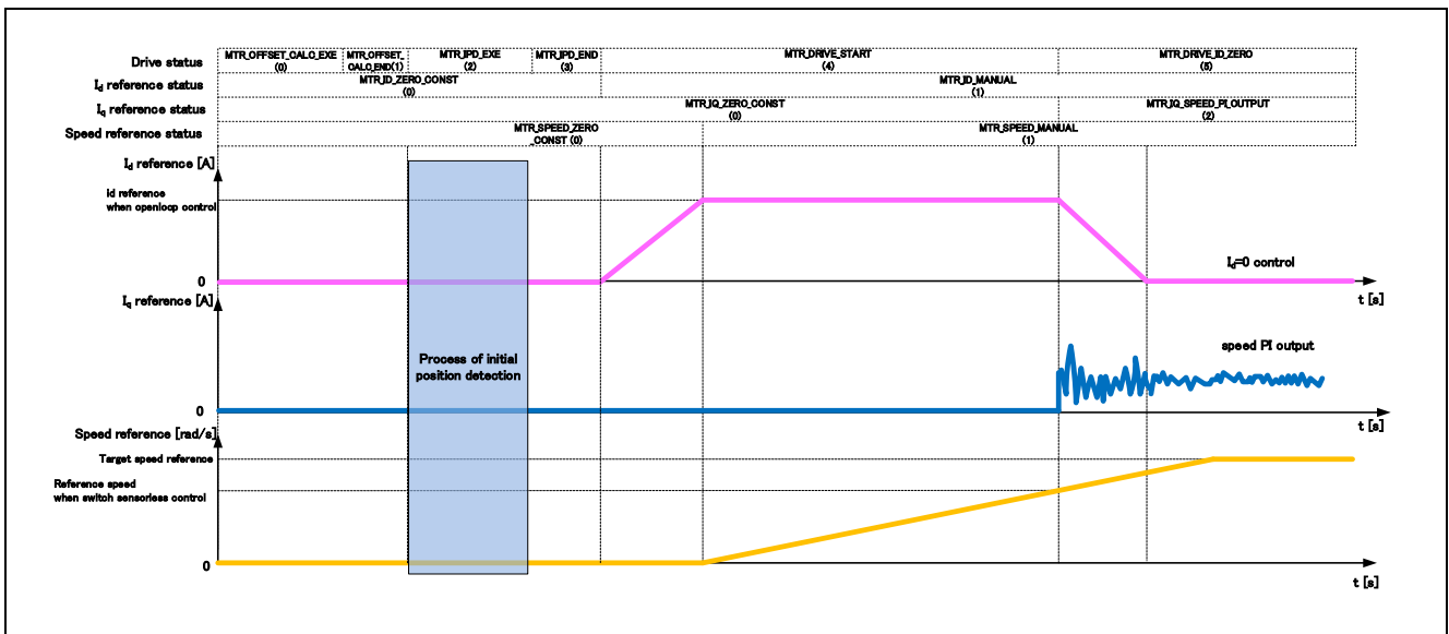
図 3-6 センサレス速度制御ソフトの始動制御内容 (IPD 処理適用)
