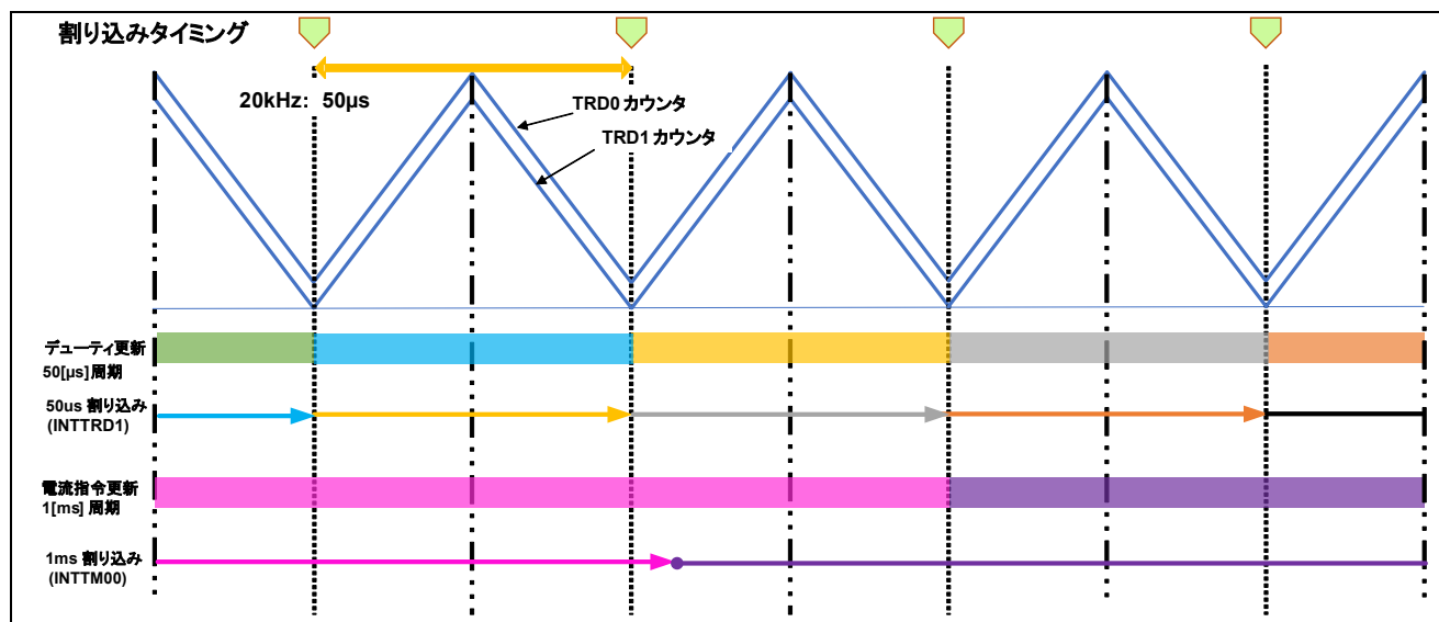
図 3-24 割り込み発生と出力値の更新イメージ
