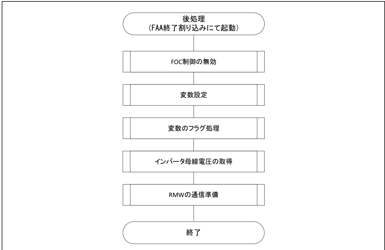
図 3-30 後処理フローチャート
