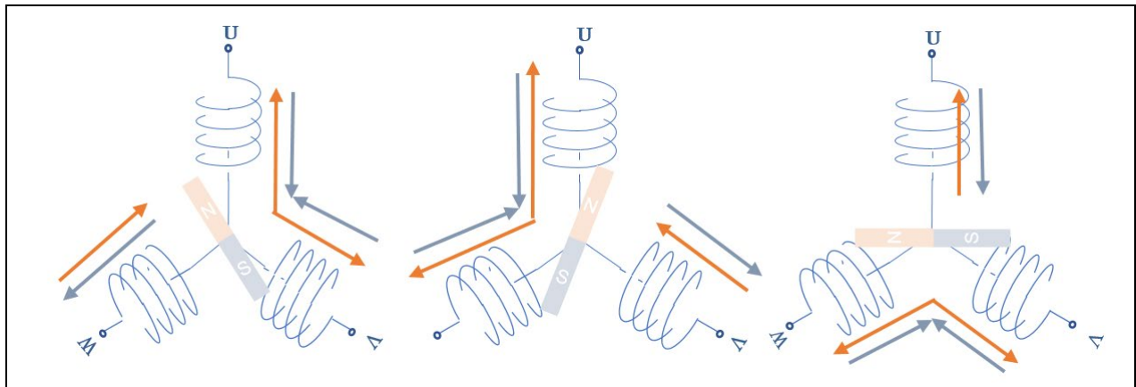
図 3-20 磁気飽和を利用した初期位置検出による電圧印加パターン例
