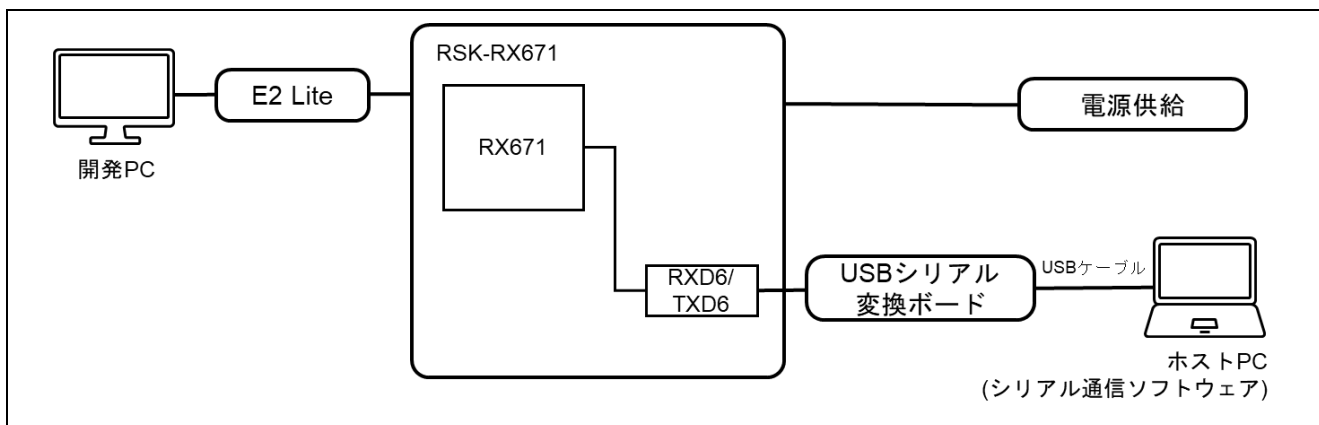
図 6-48 RSK-RX671 機器接続図
