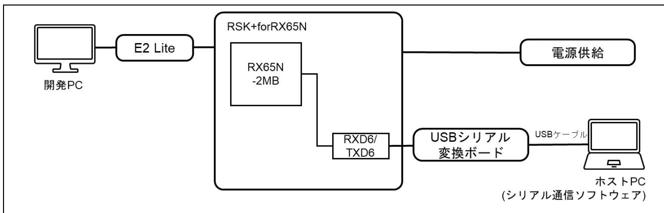
図 6-35 RSK-RX65N 機器接続図
