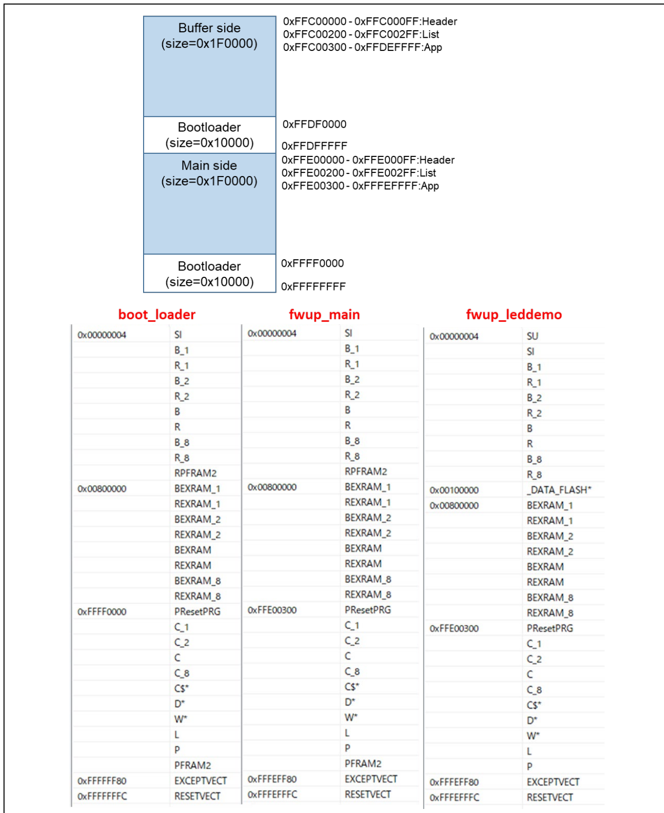
図 6-55 RX72N デュアルバンク方式のデモプロジェクトのメモリマップ
