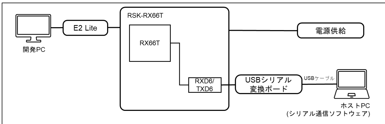
図 6-40 RSK-RX66T 機器接続図
