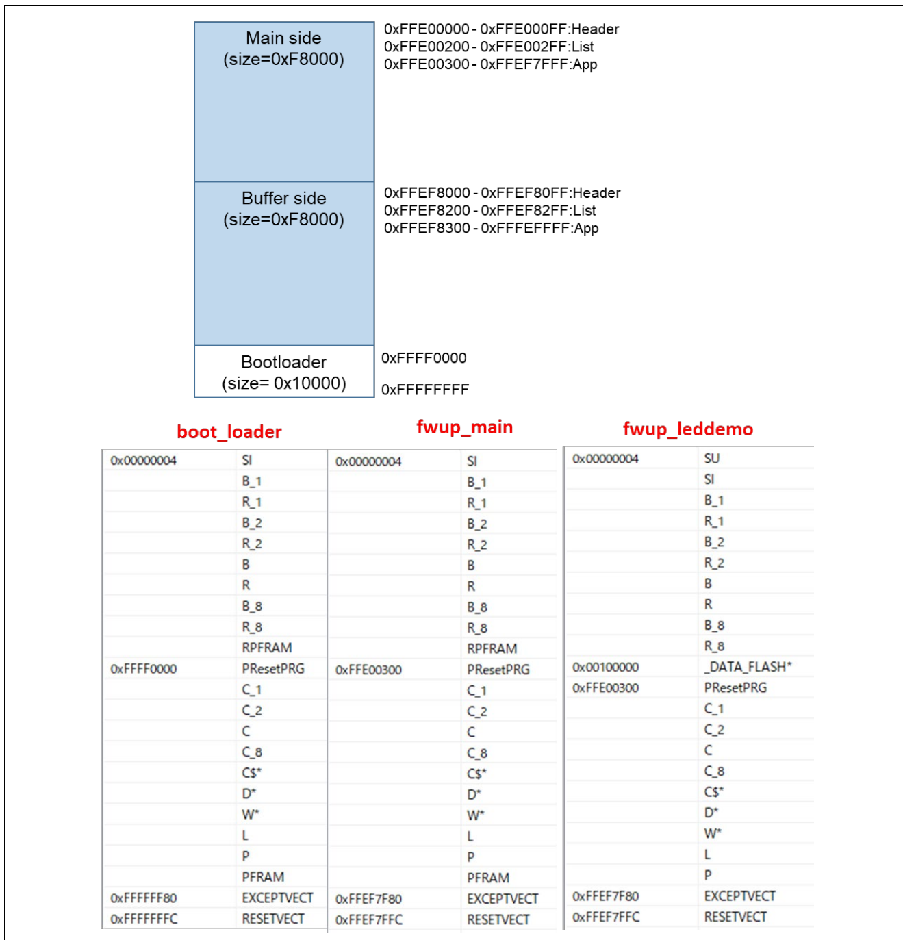
図 6-51 RX671 リニアモードの半面更新方式のデモプロジェクトのメモリマップ
