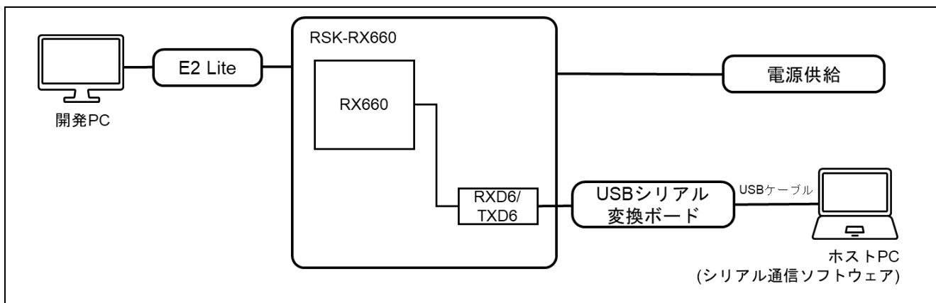
図 6-44 RSK-RX660 機器接続図
