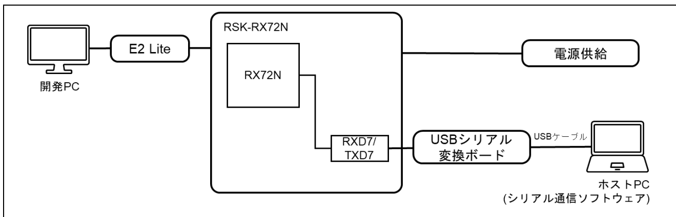
図 6-53 RSK-RX72N 機器接続図
