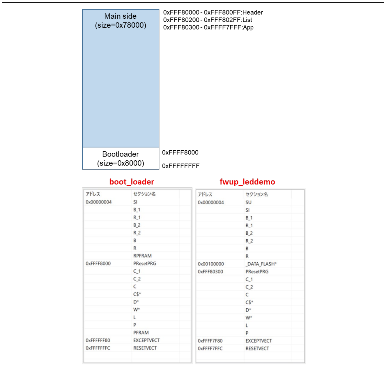
図 6-28 RX261 リニアモードの全面更新方式のデモプロジェクトのメモリマップ
