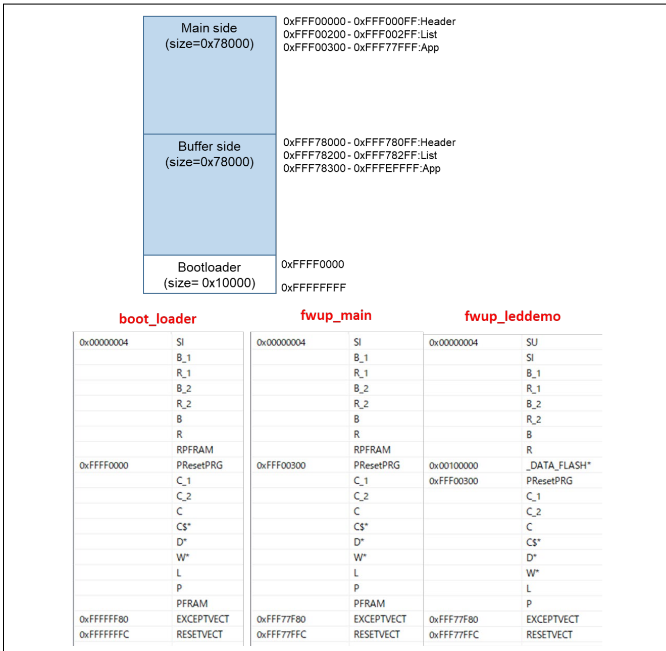
図 6-46 RX660 リニアモードの半面更新方式のデモプロジェクトのメモリマップ
