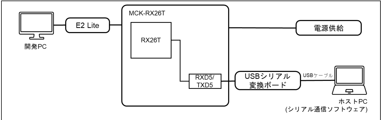
図 6-29 MCK-RX26T 機器接続図
