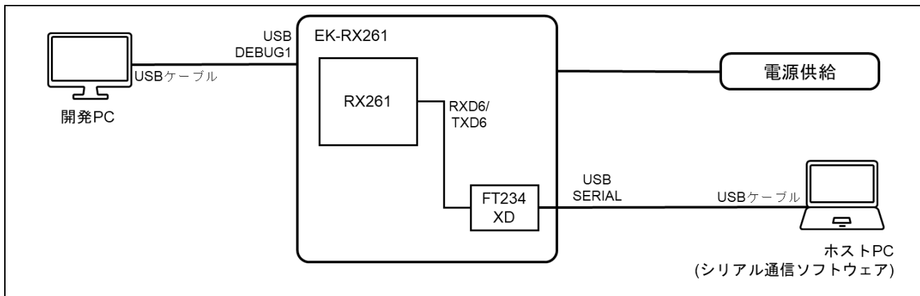
図 6-25 EK-RX261 機器接続図
