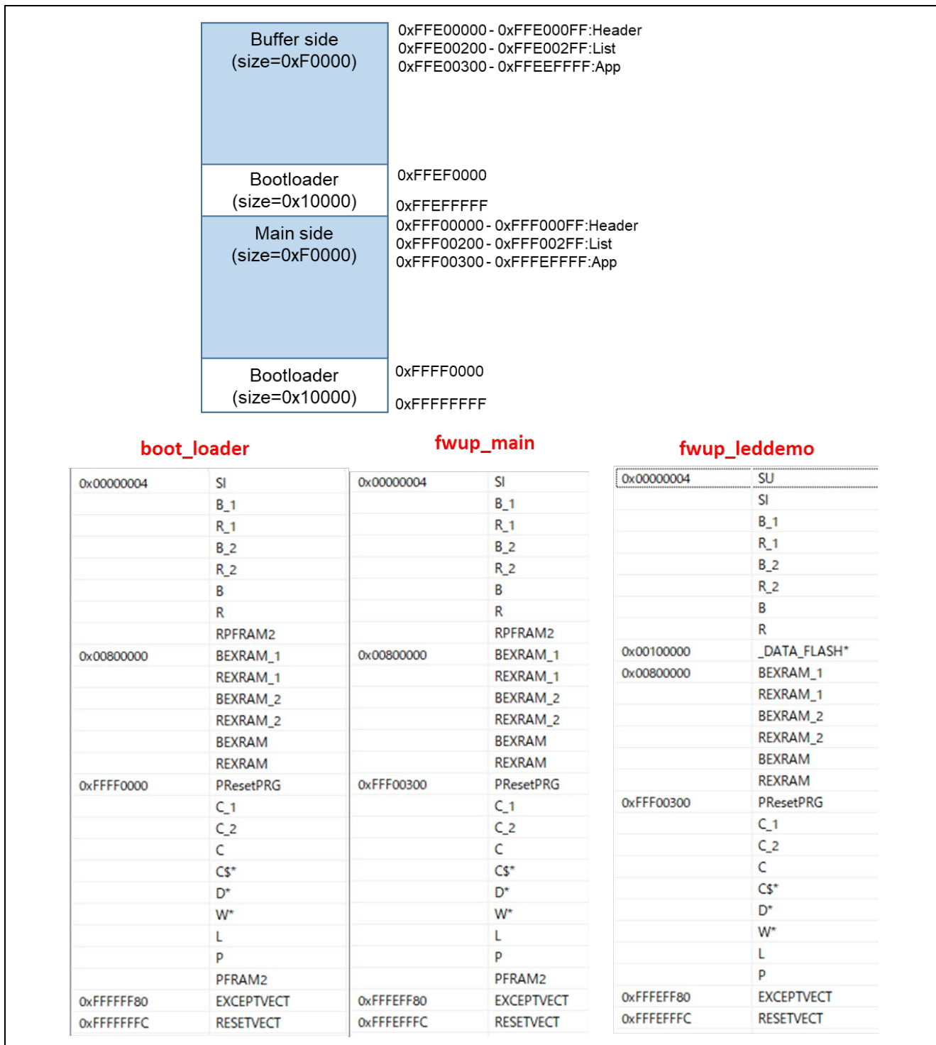
図 6-37 RX65N デュアルバンク方式のデモプロジェクトのメモリマップ
