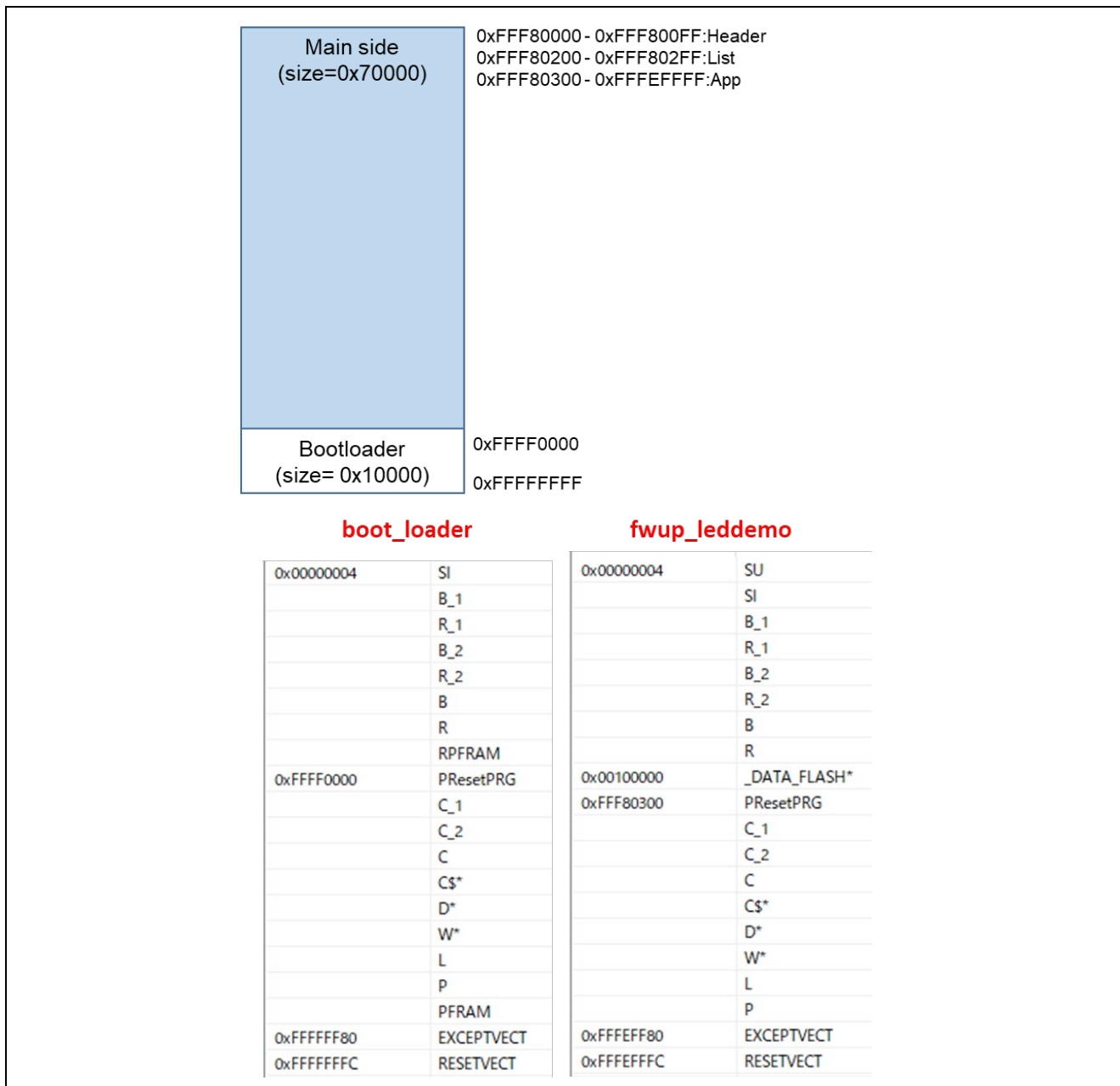
図 6-43 RX66T リニアモードの全面更新方式のデモプロジェクトのメモリマップ
