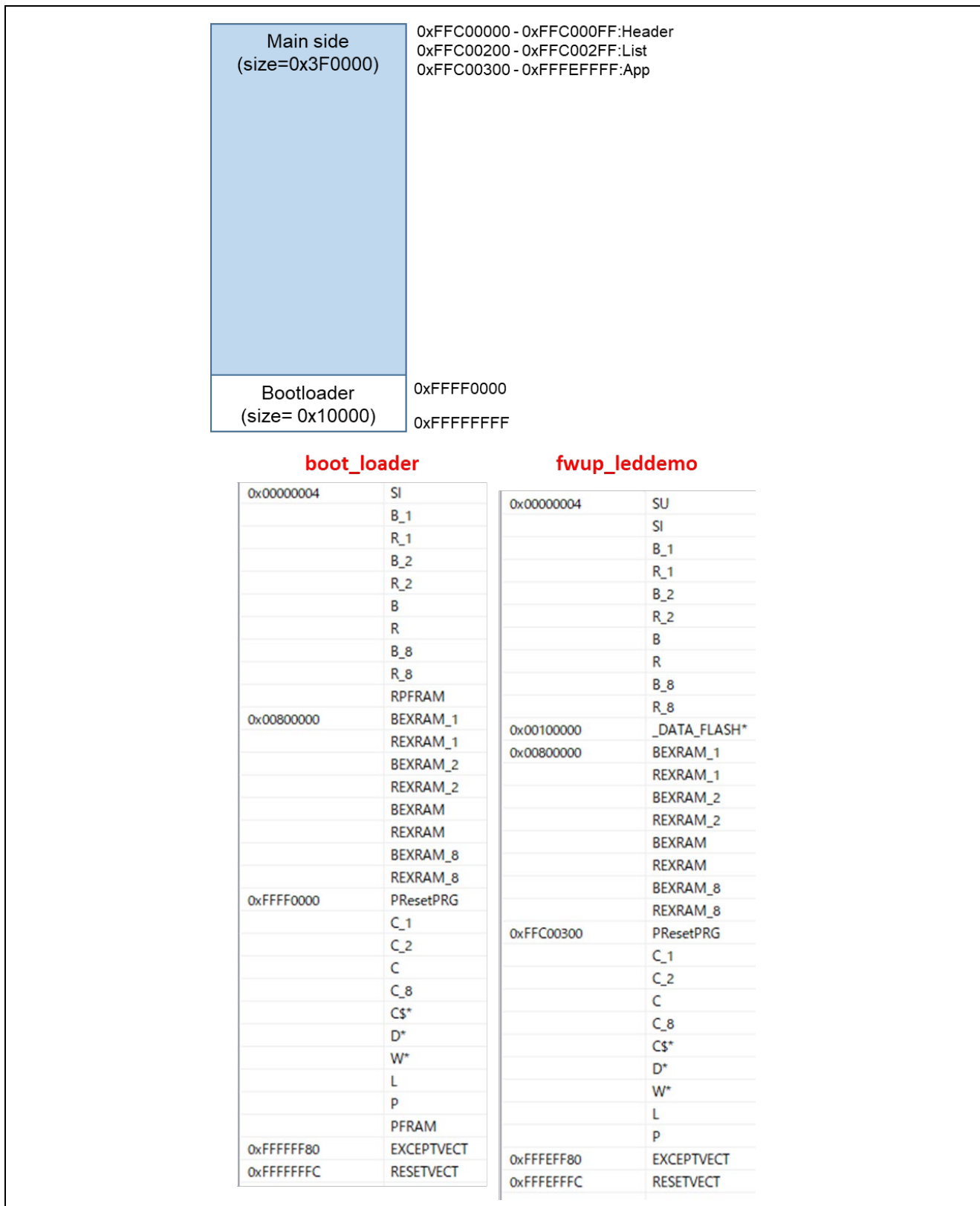
図 6-57 RX72N リニアモードの全面更新方式のデモプロジェクトのメモリマップ
