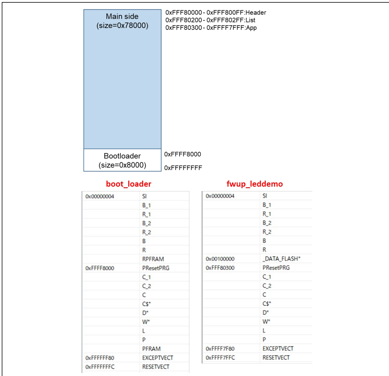
図 6-34 RX26T リニアモードの全面更新方式のデモプロジェクトのメモリマップ
