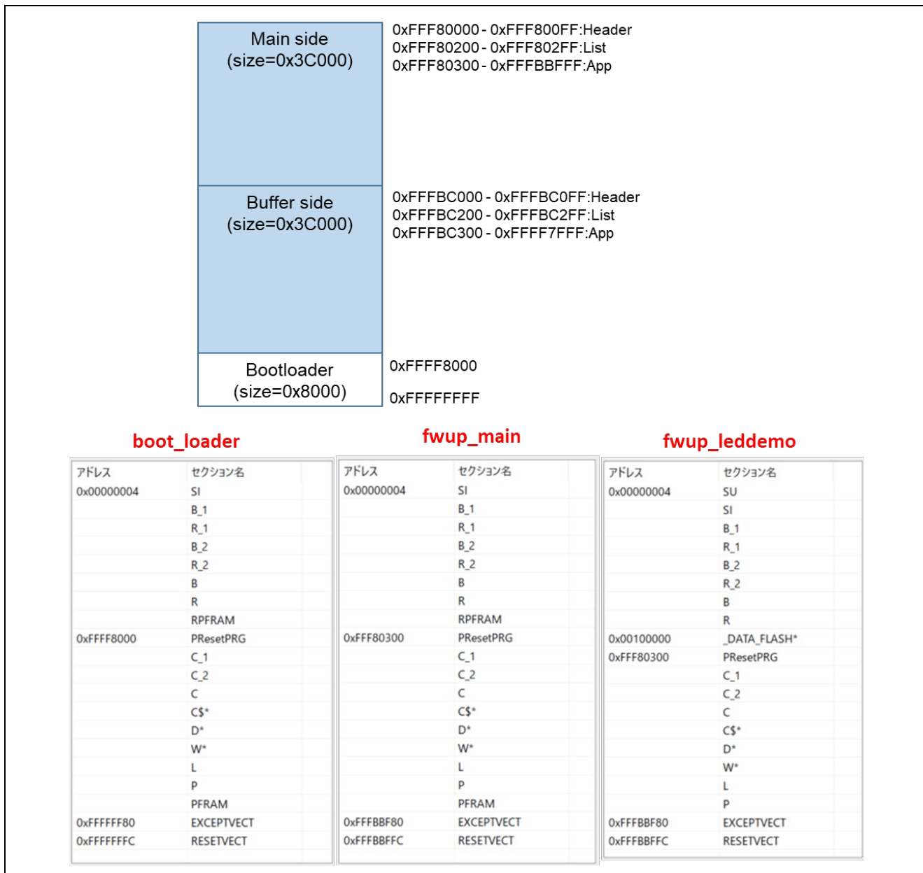
図 6-27 RX261 リニアモードの半面更新方式のデモプロジェクトのメモリマップ
