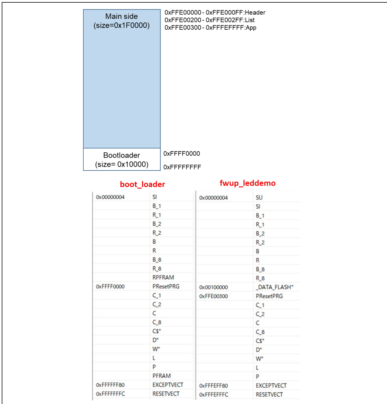
図 6-52 RX671 リニアモードの全面更新方式のデモプロジェクトのメモリマップ
