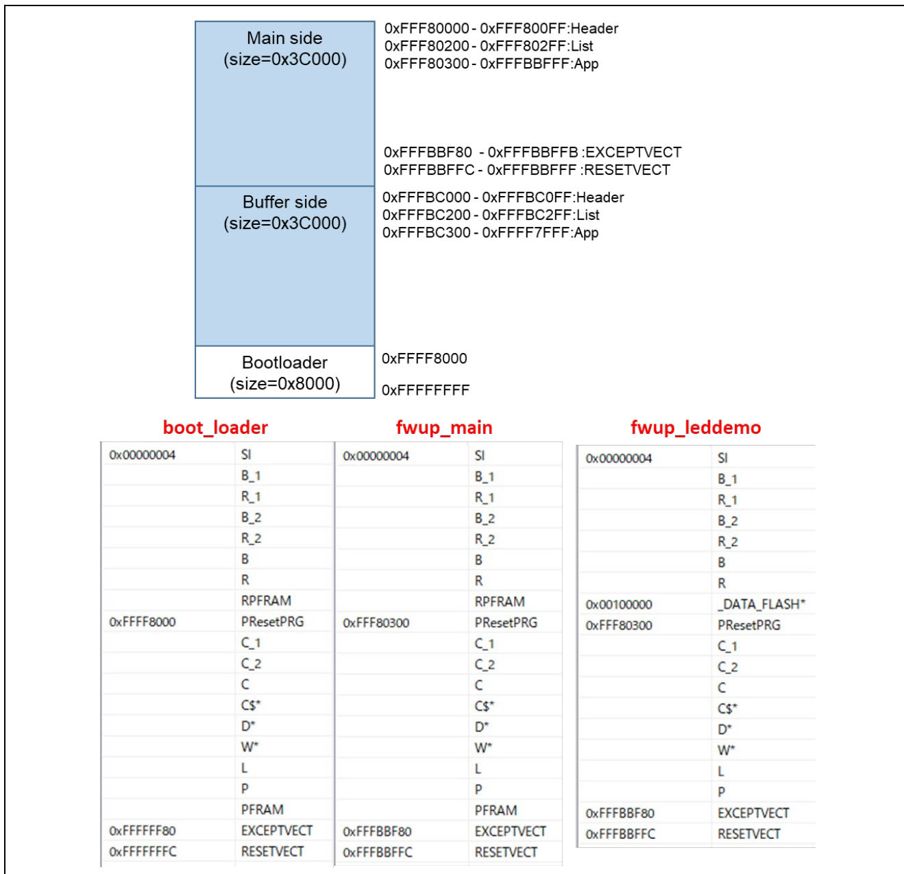
図 6-33 RX26T リニアモードの半面更新方式のデモプロジェクトのメモリマップ
