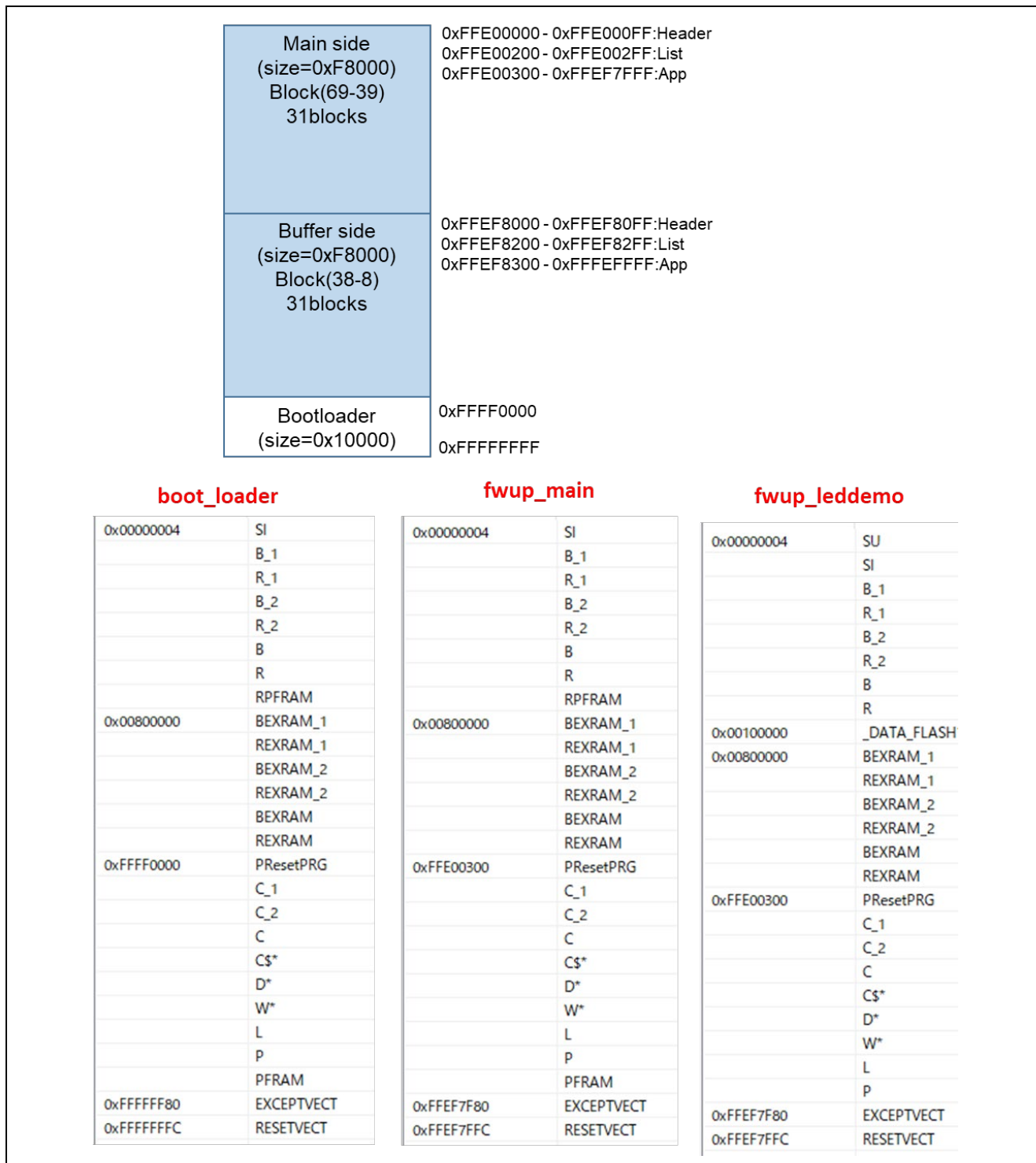
図 6-38 RX65N リニアモードの半面更新方式のデモプロジェクトのメモリマップ
