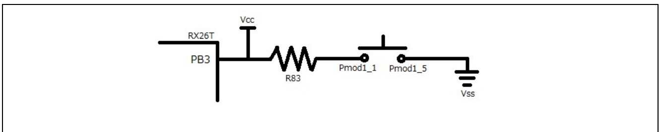
図 6-31 MCK-RX26T 外部接続 SW
