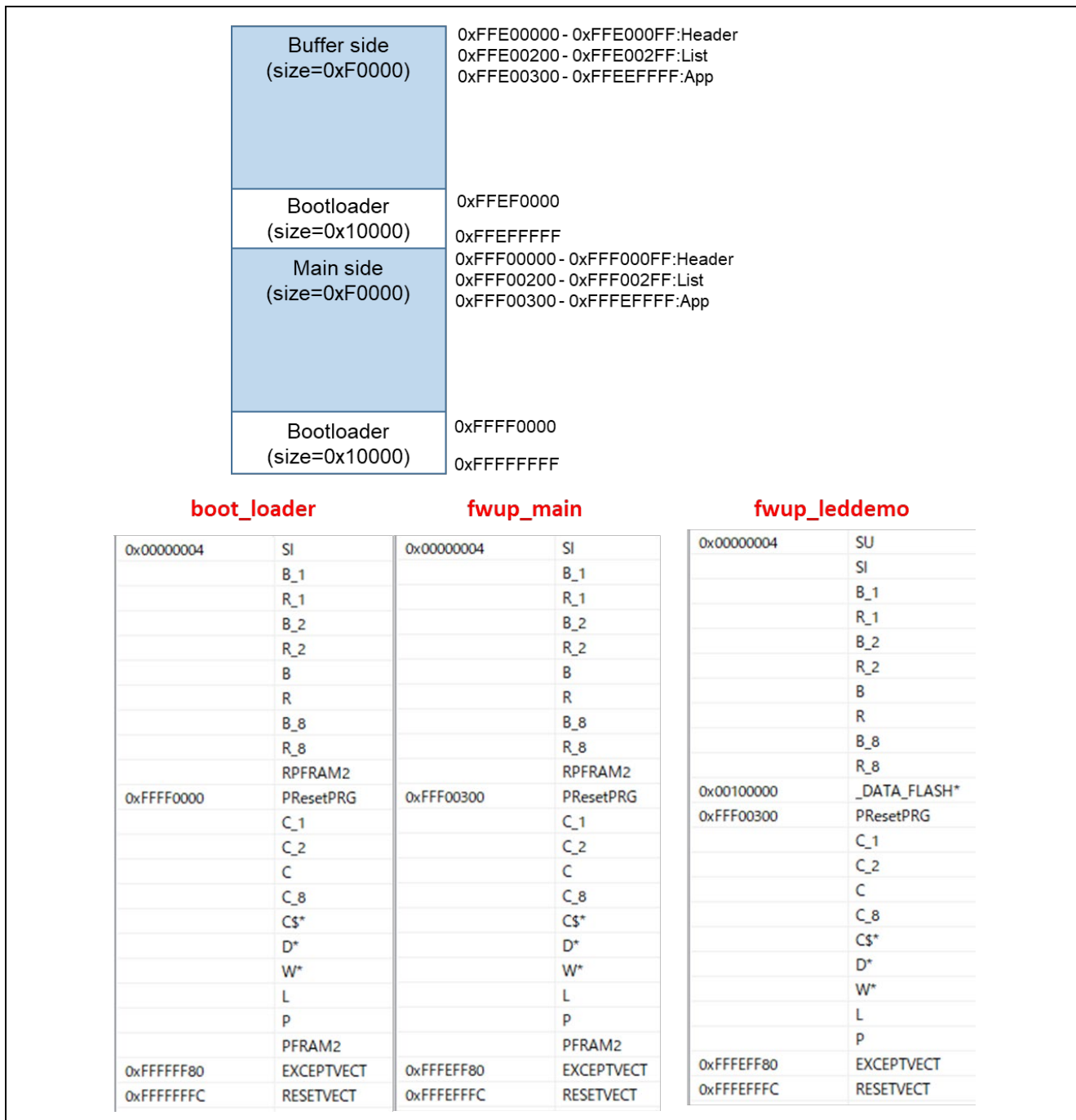
図 6-50 RX671 デュアルバンク方式のデモプロジェクトのメモリマップ
