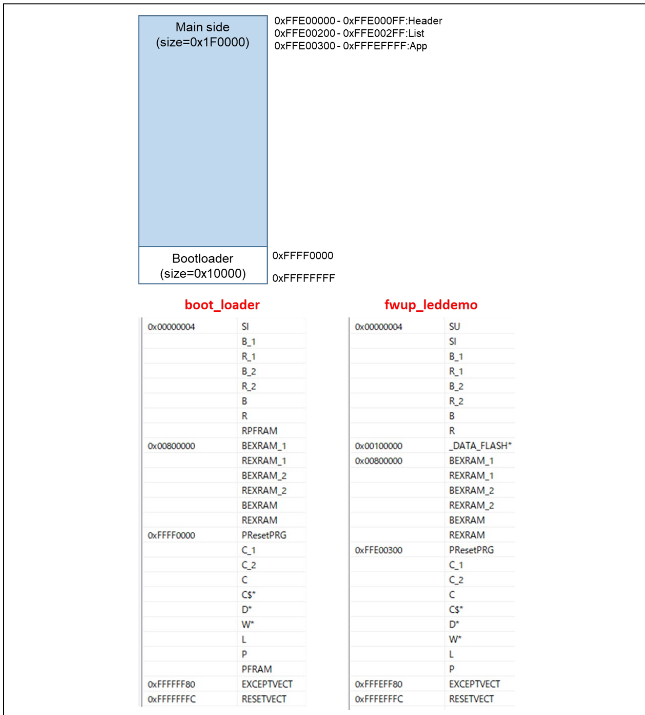
図 6-39 RX65N リニアモードの全面更新方式のデモプロジェクトのメモリマップ
