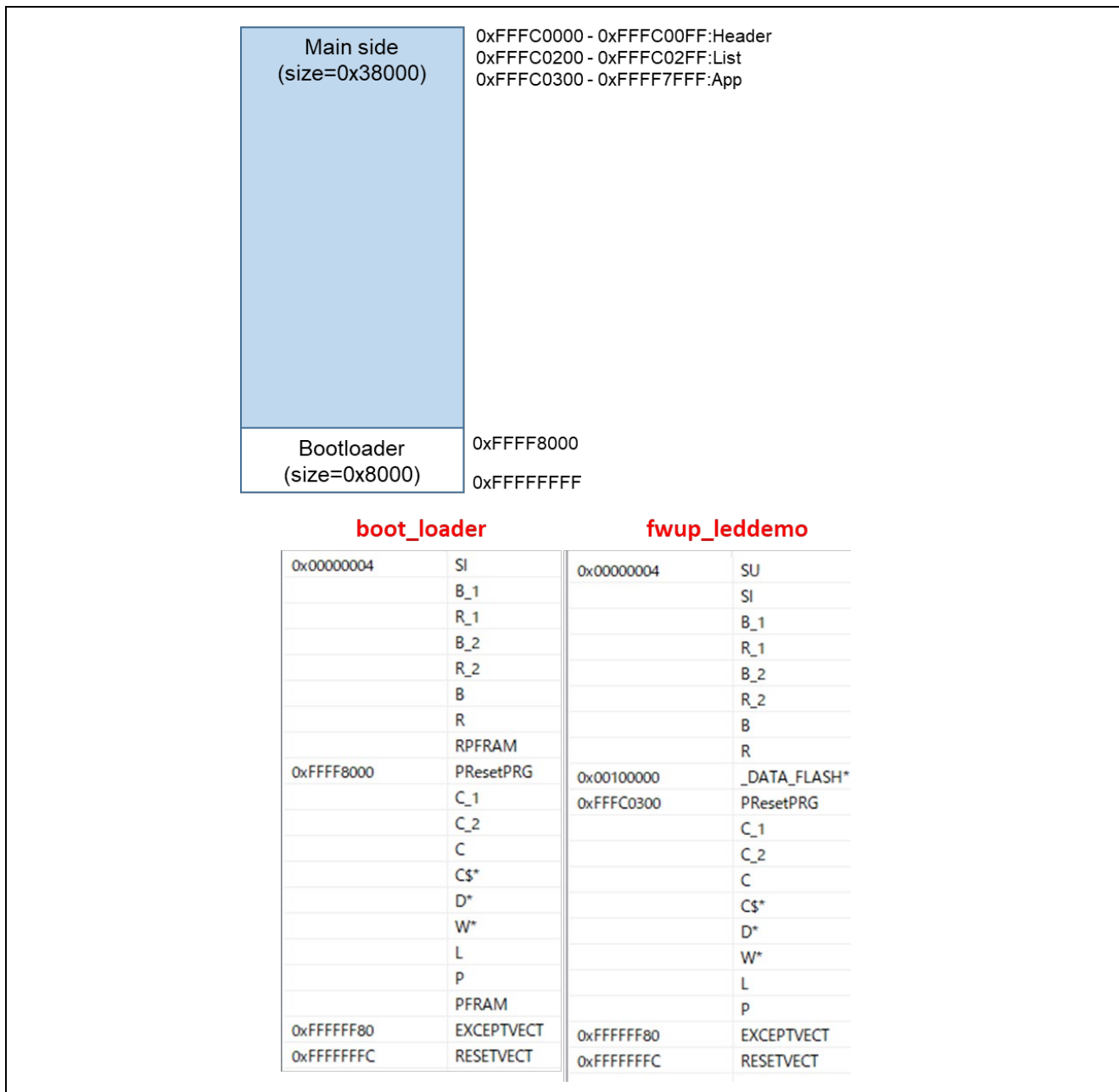
図 6-20 RX23E-B リニアモードの全面更新方式のデモプロジェクトのメモリマップ
