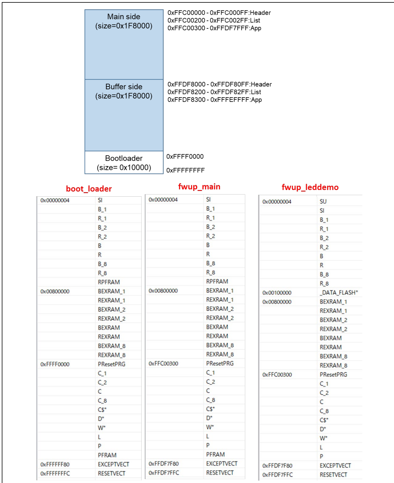
図 6-56 RX72N リニアモードの半面更新方式のデモプロジェクトのメモリマップ
