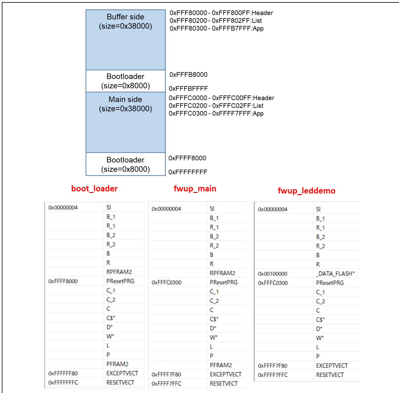
図 6-32 RX26T デュアルバンク方式のデモプロジェクトのメモリマップ
