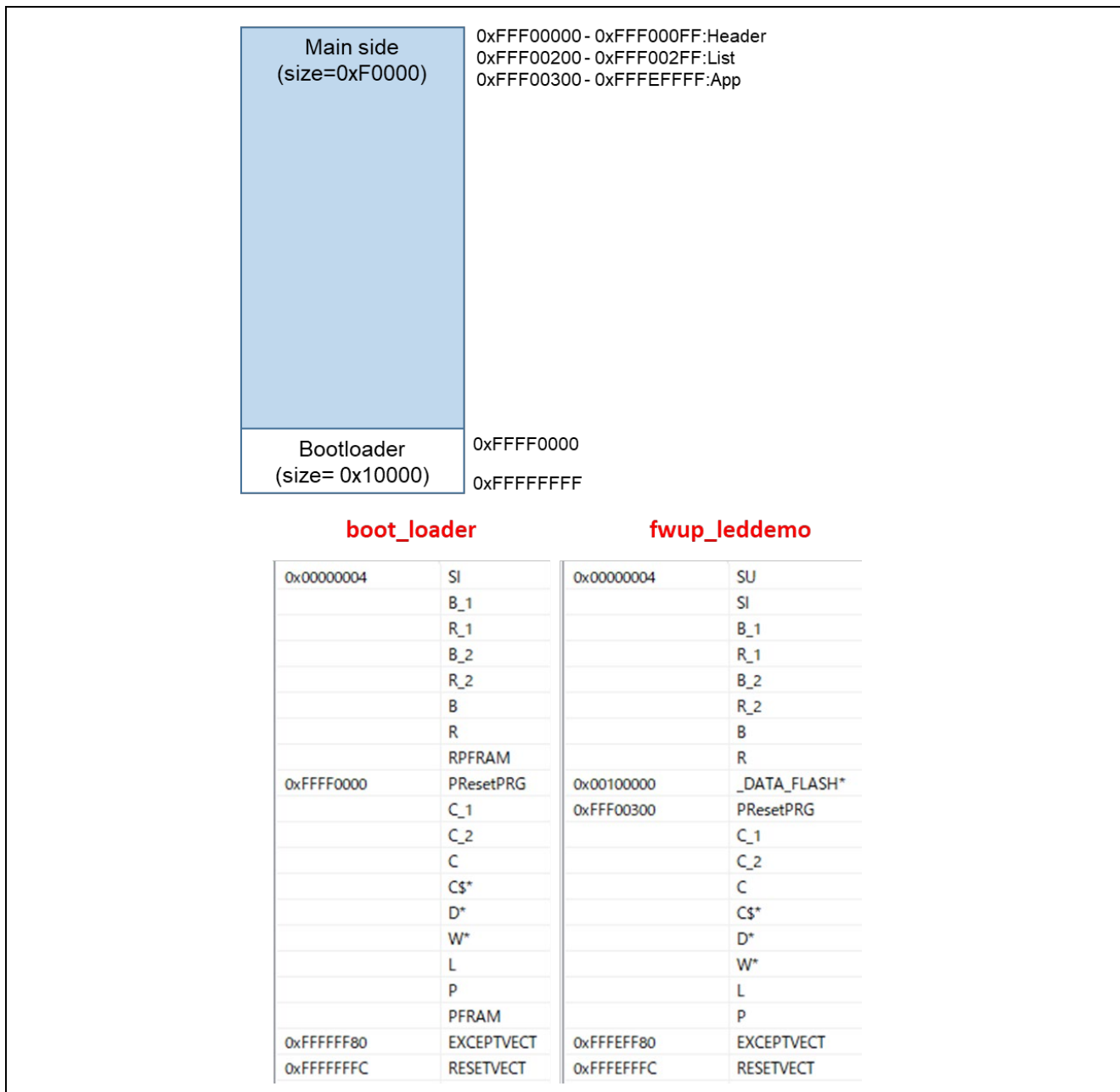
図 6-47 RX660 リニアモードの全面更新方式のデモプロジェクトのメモリマップ
