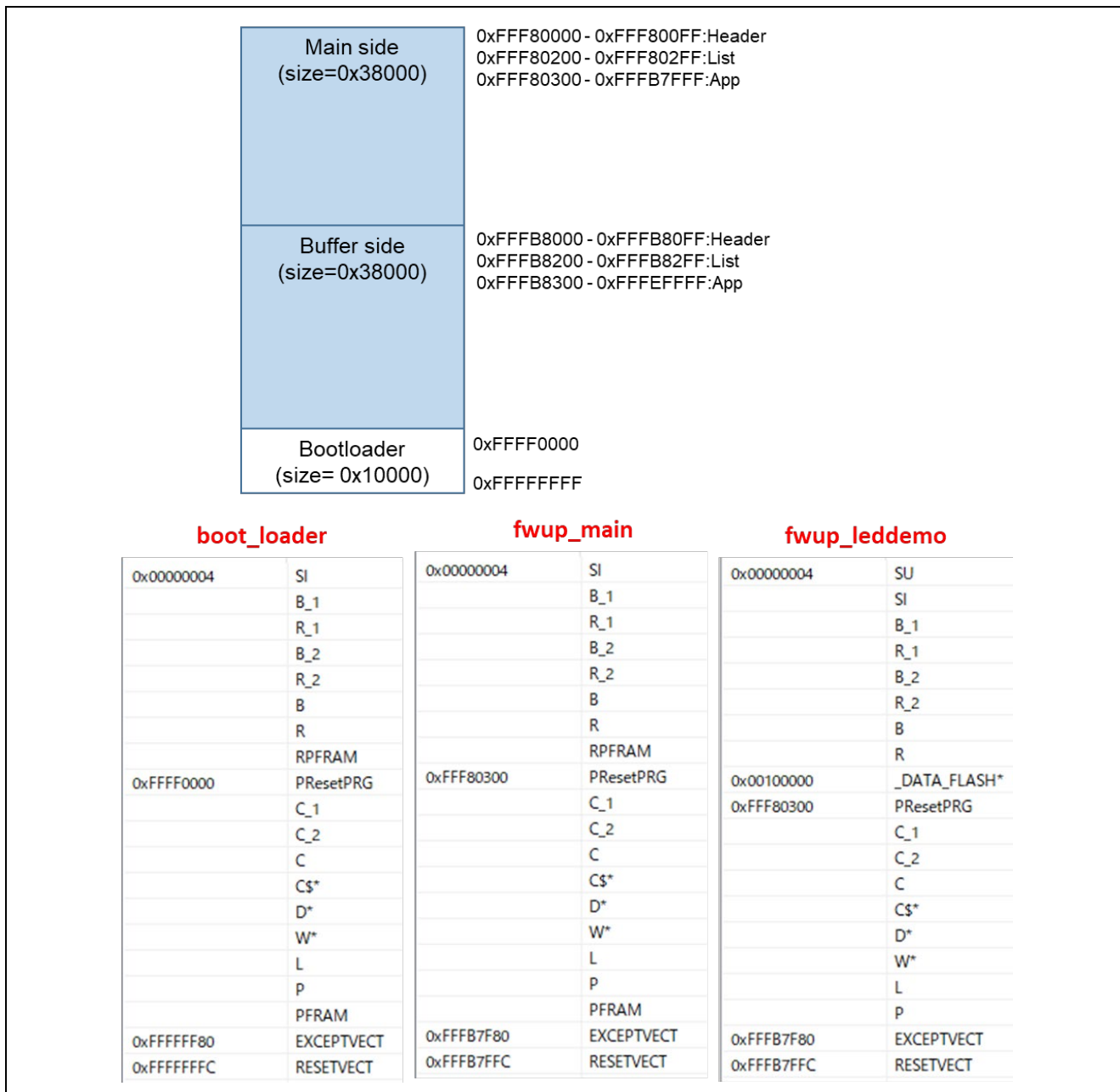
図 6-42 RX66T リニアモードの半面更新方式のデモプロジェクトのメモリマップ
