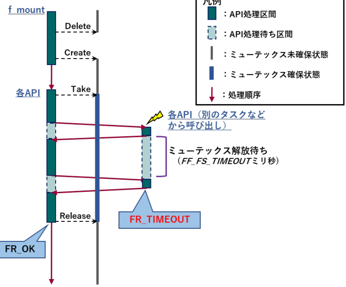
図 1.2 ボリュームに対する排他制御
