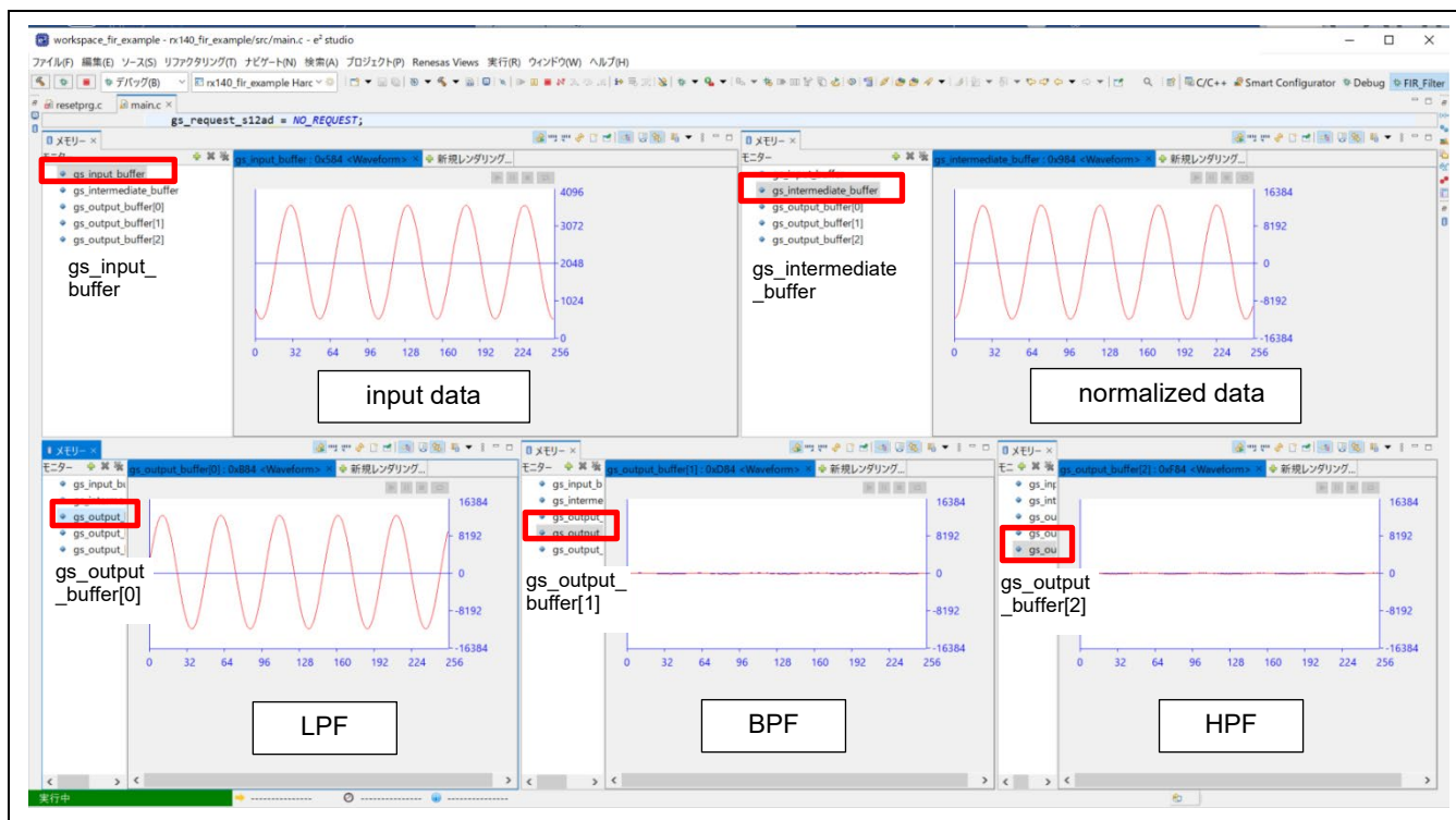
図 2.5 FIR_Filter パースペクティブ
