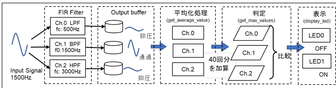
図 3.7 周波数帯域判定のイメージ
