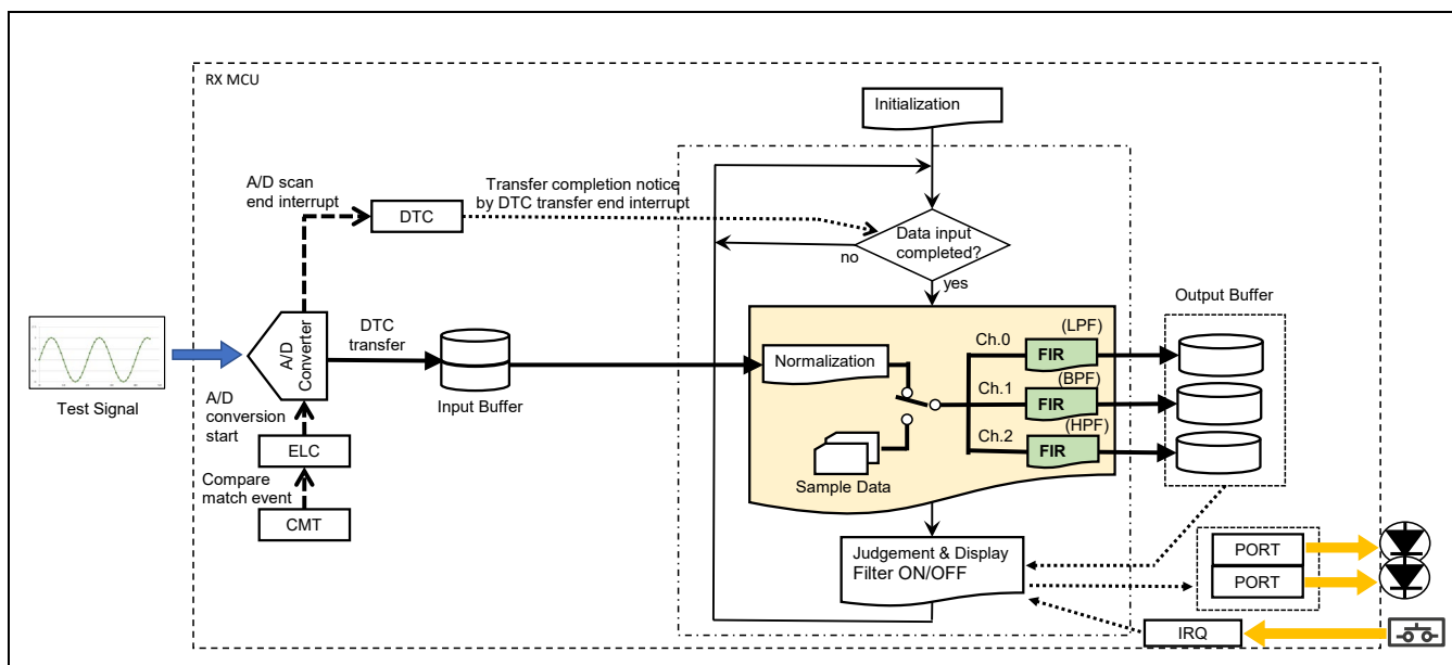
図 1.1 システムの概要
