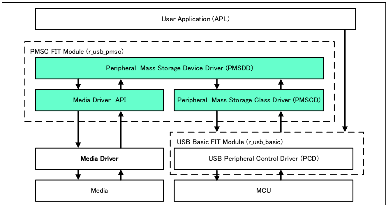
Figure 2-1 モジュール構成図
