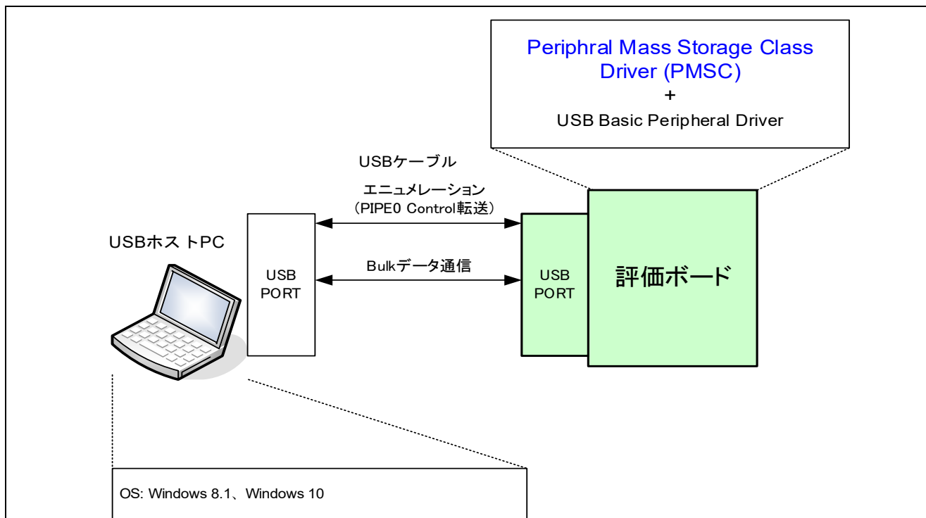
Figure 4-1 PMSC動作環境例
