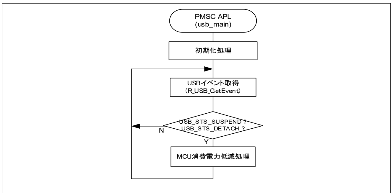
Figure 4-3 APL 処理概要
