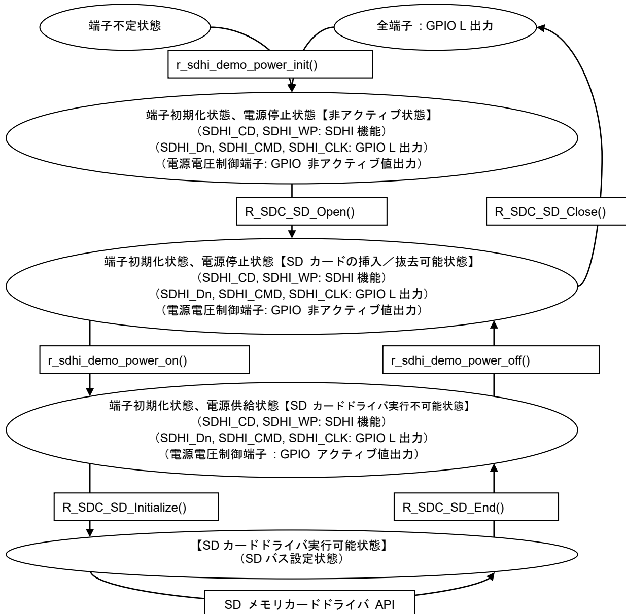
図 5-1 状態遷移図
