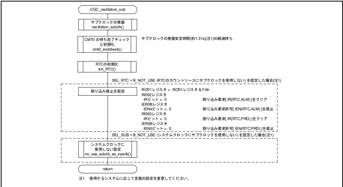
図4.8 サブクロックの発振設定
