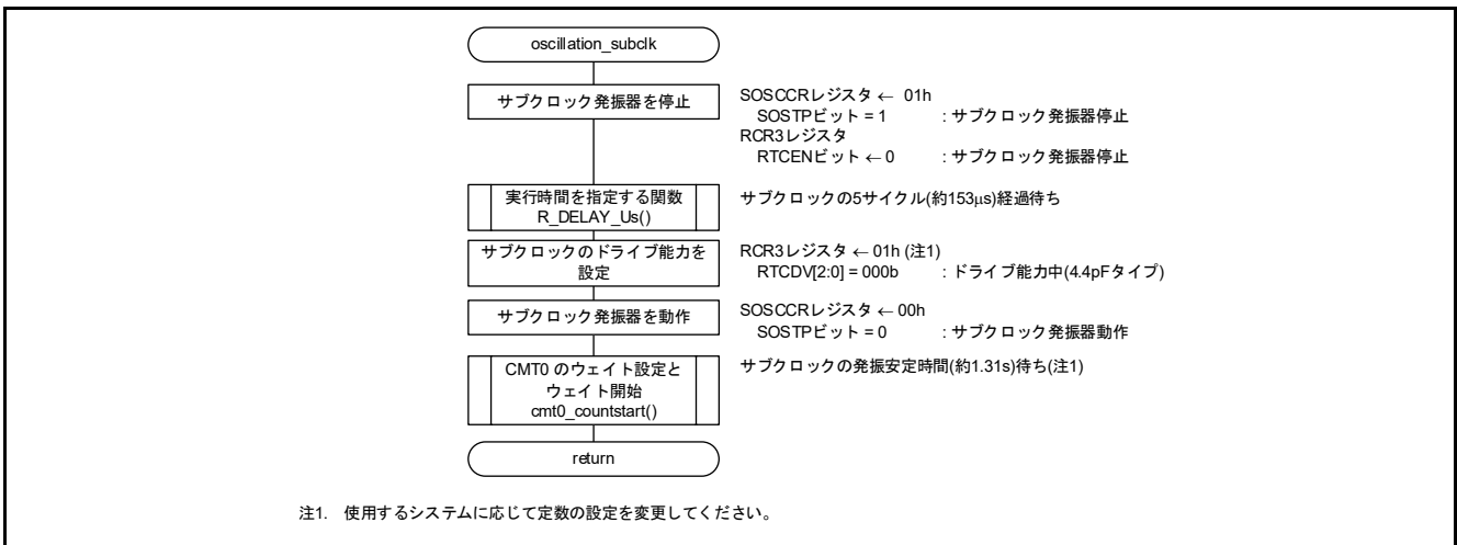
図4.9 サブクロックの発振
