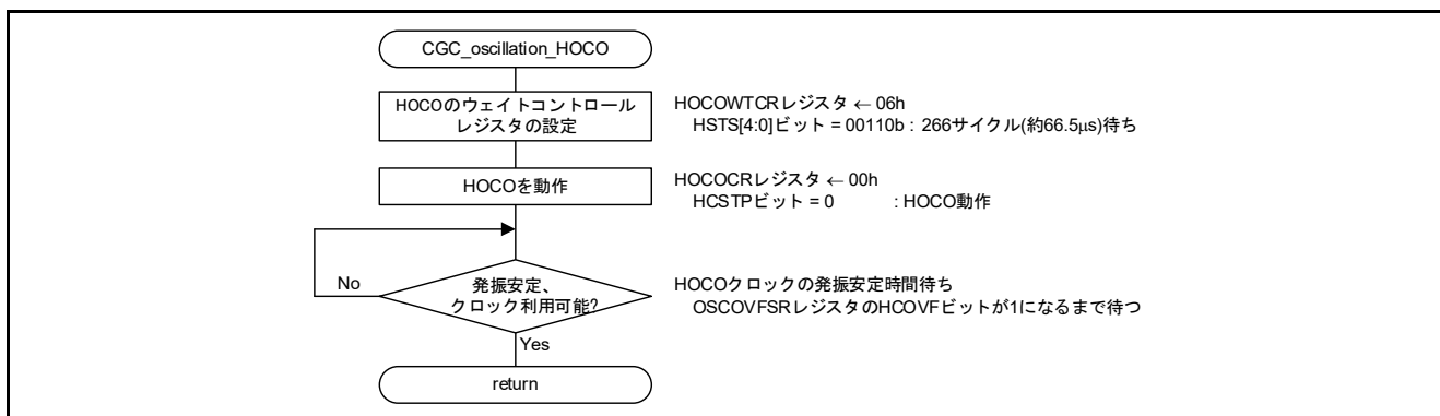
図4.7 HOCO クロックの発振設定
