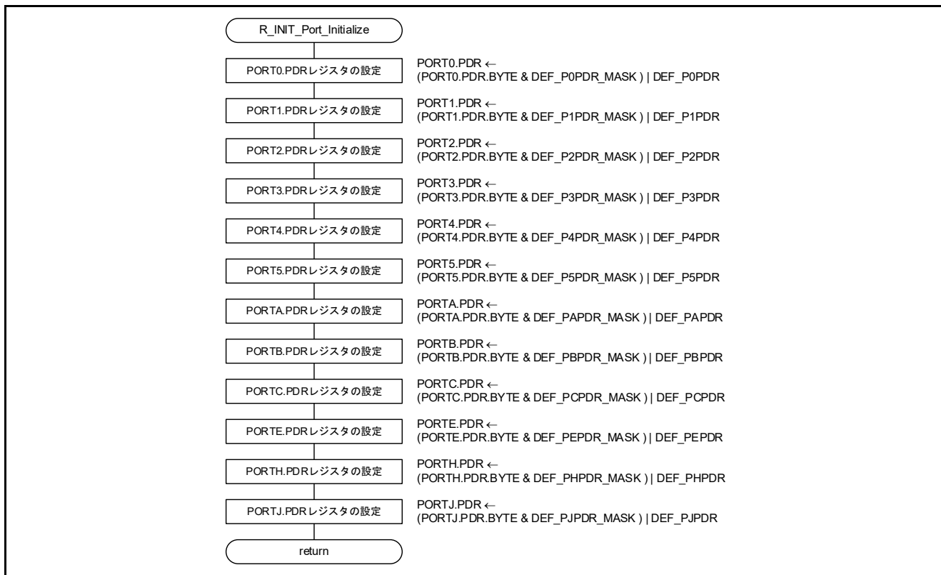
図4.4 存在しないポートの初期設定
