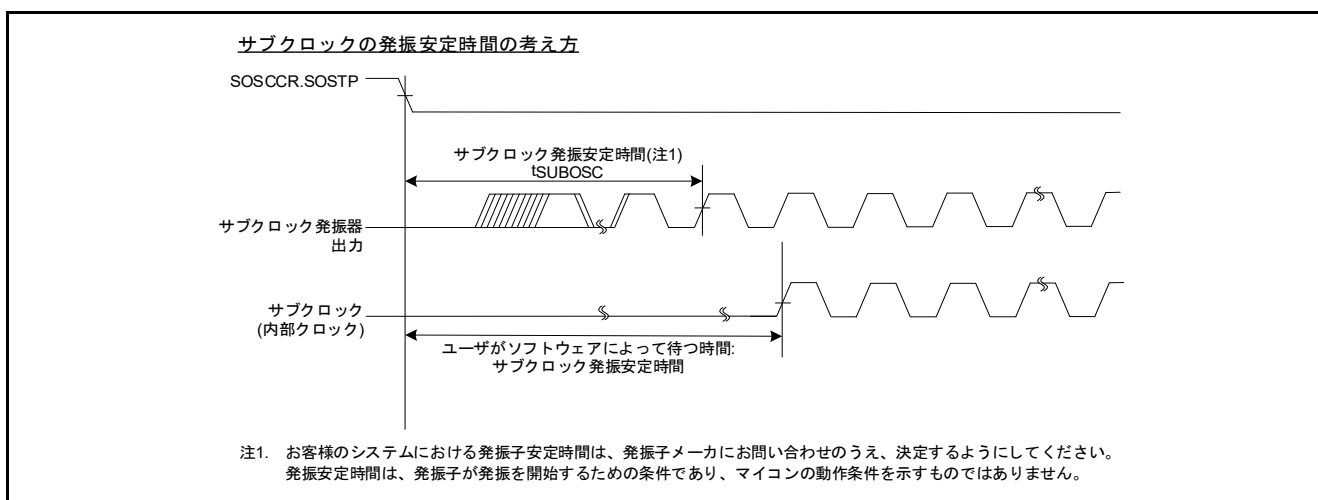
図4.1 サブクロックの発振安定時間の考え方
