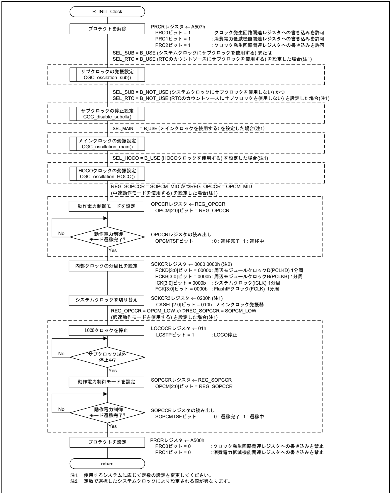
図4.5 クロック初期設定
