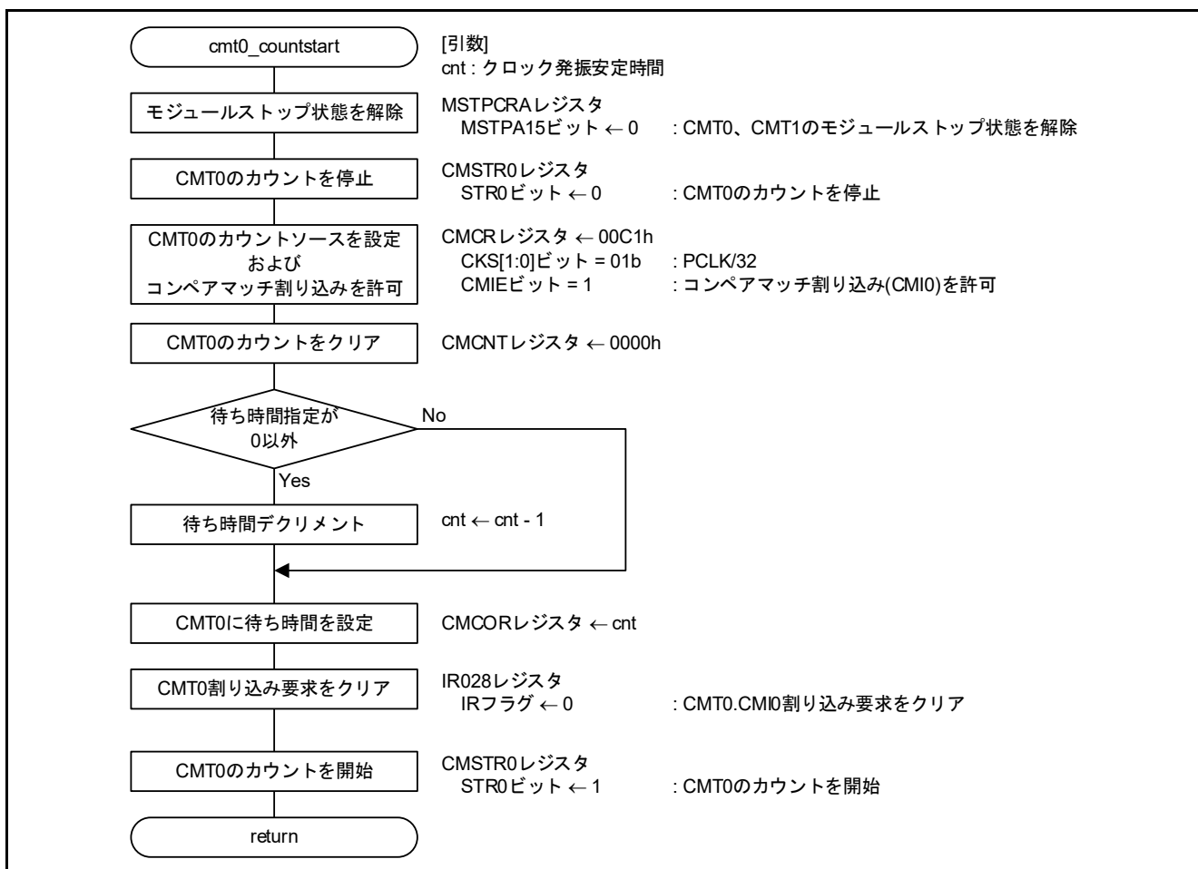
図4.13 CMT0の待ち開始設定
