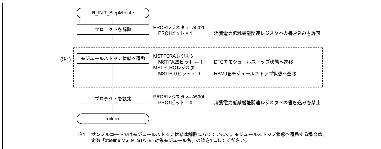
図4.3 リセット後に動作している周辺機能の停止
