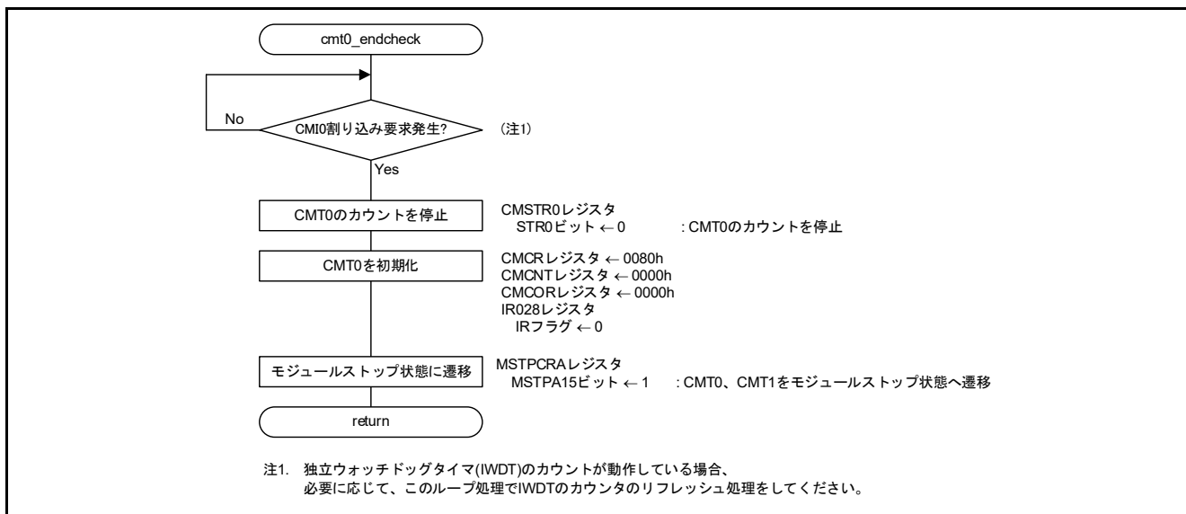
図4.14 CMT0 の待ち完了チェックと初期化
