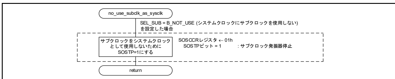
図4.11 サブクロックをシステムクロックとして使用しない場合の設定
