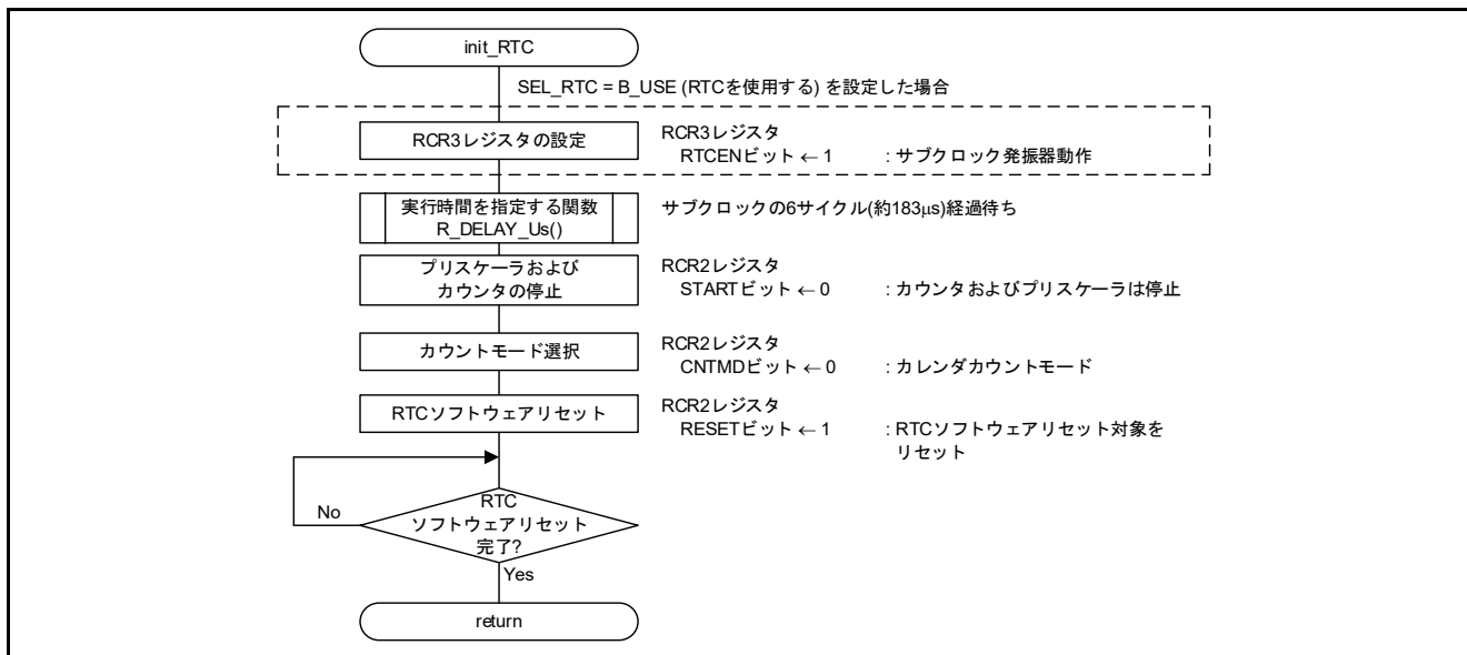
図4.10 RTCの初期化
