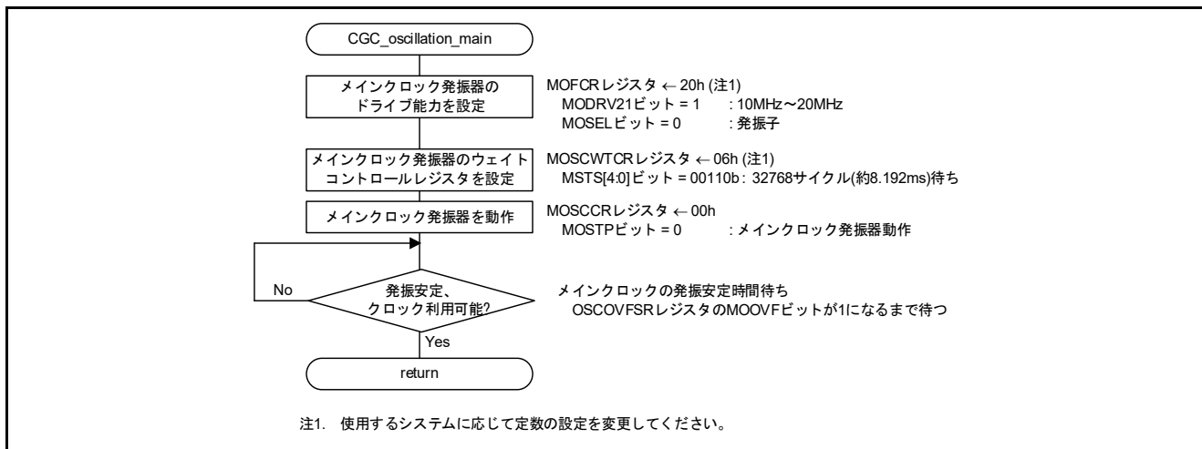
図4.6 メインクロックの発振設定
