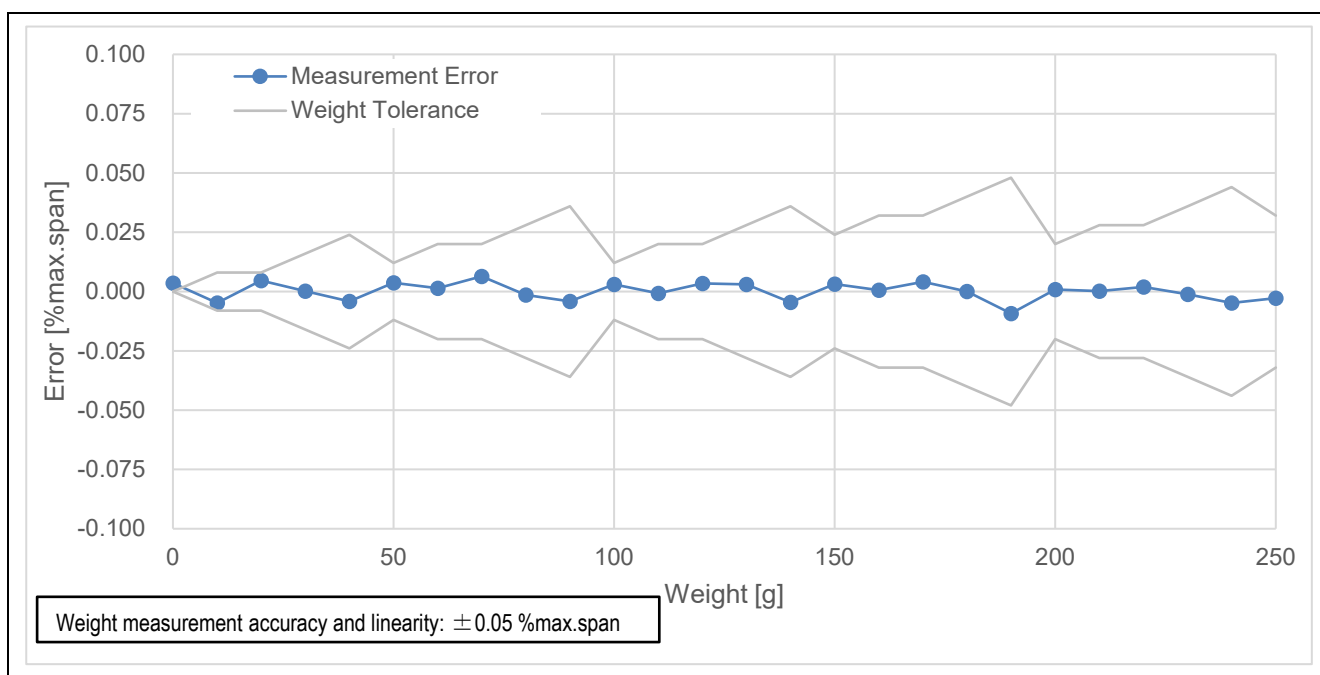
図 3-2 重量計測誤差（周囲温度：25°C）
