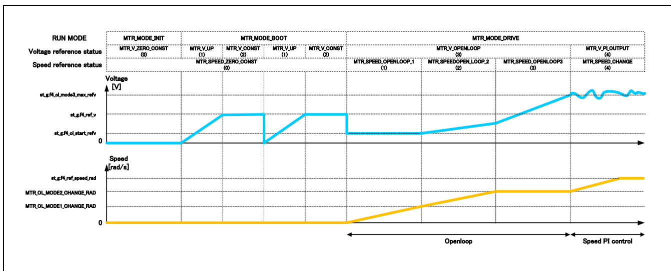
図 3-6 始動方法例
