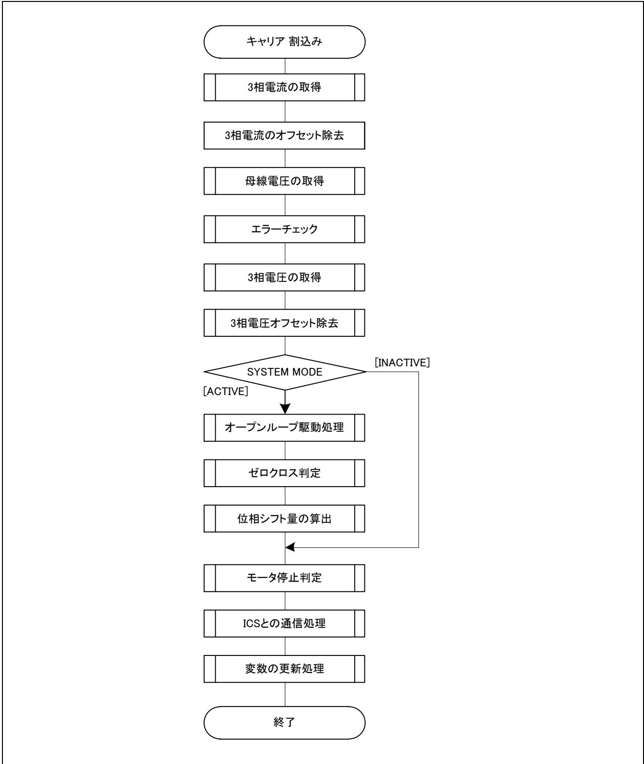
図 3-8 50 [μs]周期割り込み処理フローチャート
