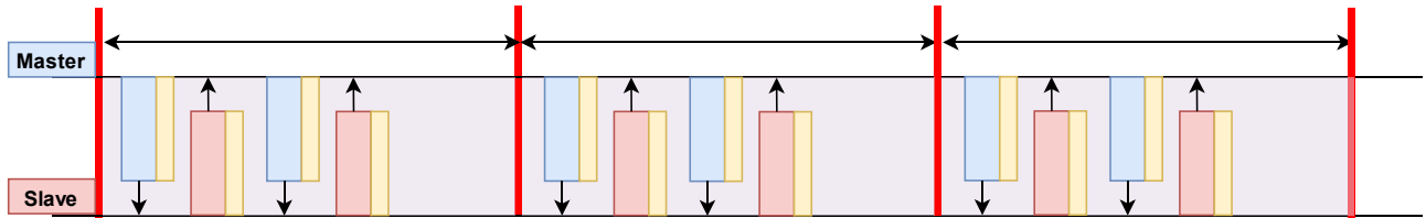
図 3.10 暗号化通信時の Link Layer の模式図
