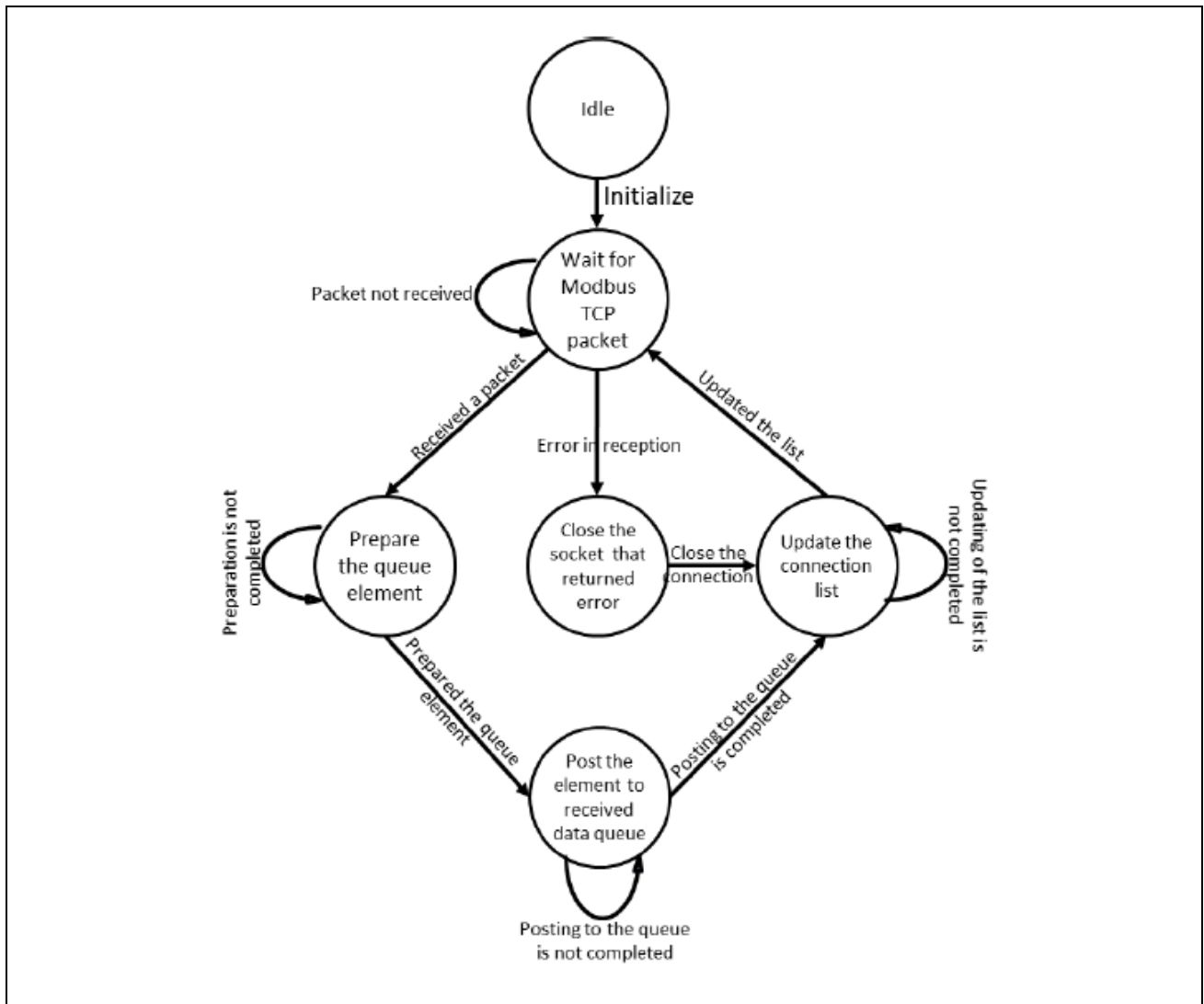
図 8.6 Modbus TCP 受信データタスク (Modbus_tcp_rcv_data_task)
