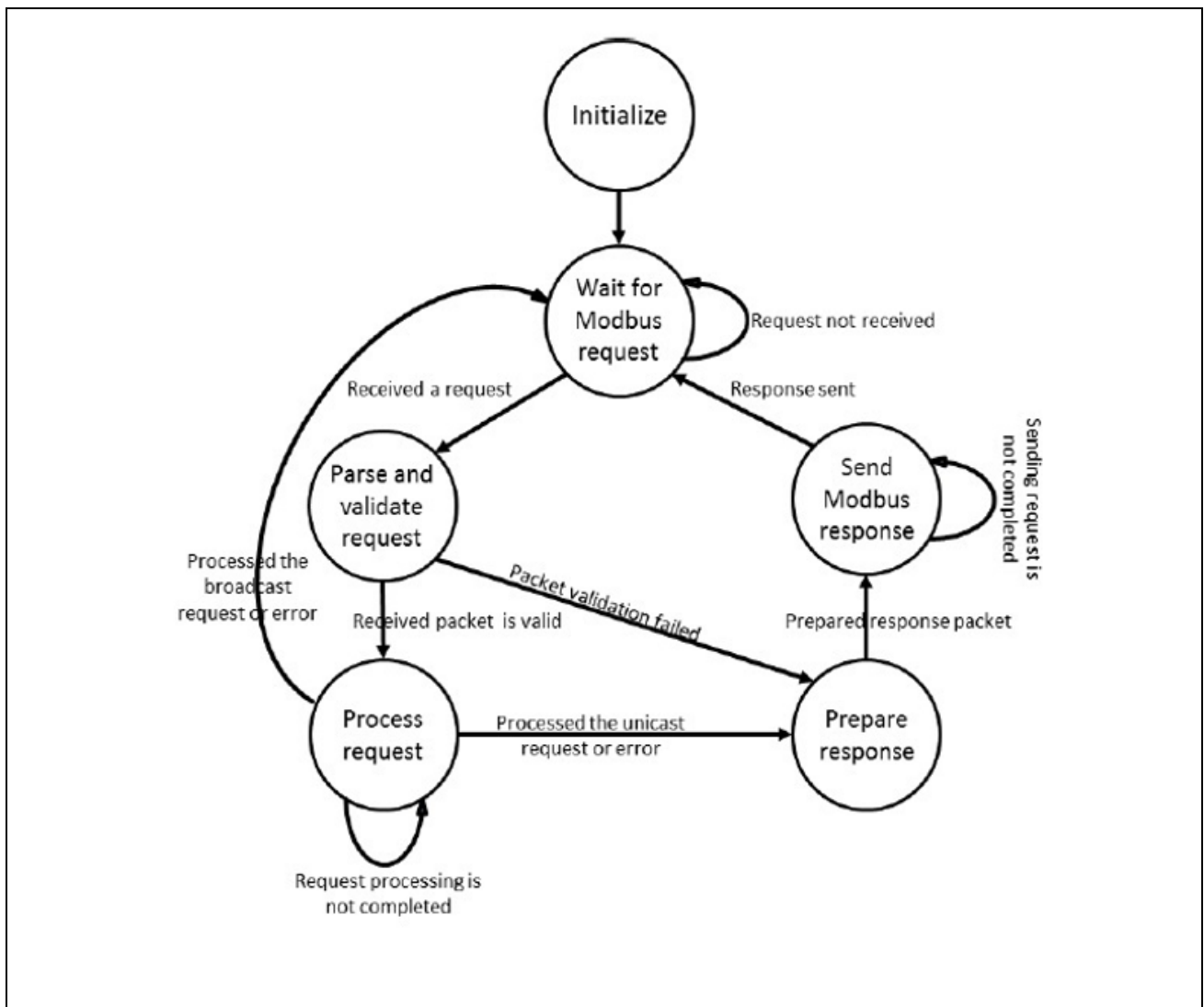
図 9.2スレーブモード時の Modbus シリアルタスク関数の状態遷移図
