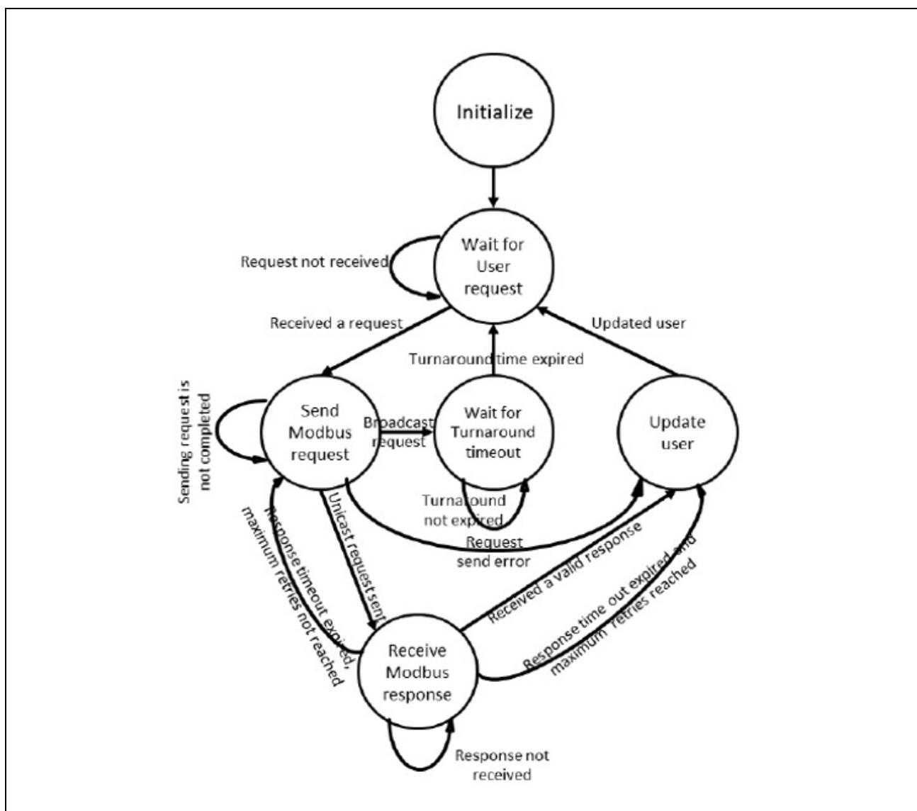
図 9.3 マスタモード時の Modbus シリアルタスク関数の状態遷移図
