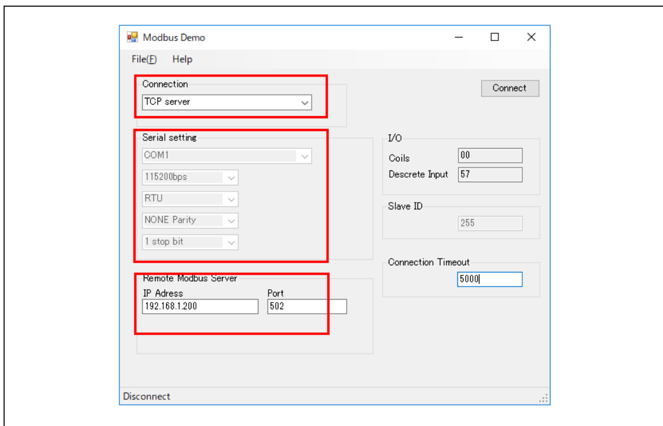
図 5.8 評価用ツール画面
