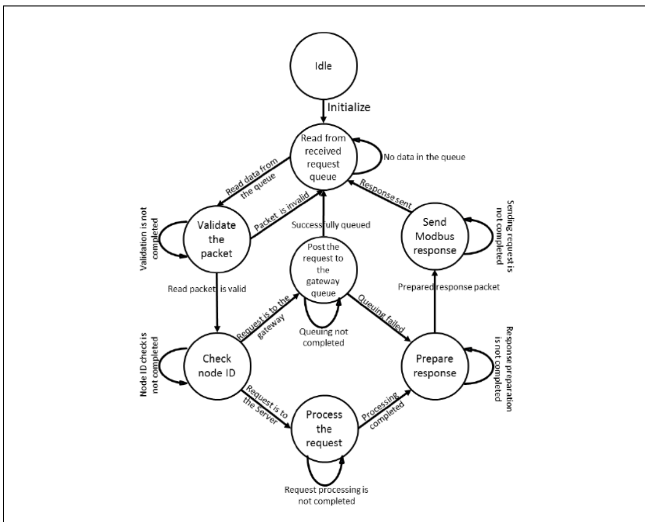
図 8.3 Modbus TCP サーバタスク (ゲートウェイ機能あり)
