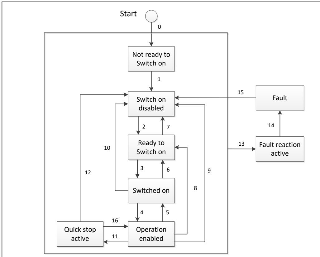
図 6-2 CiA402 状態遷移図
