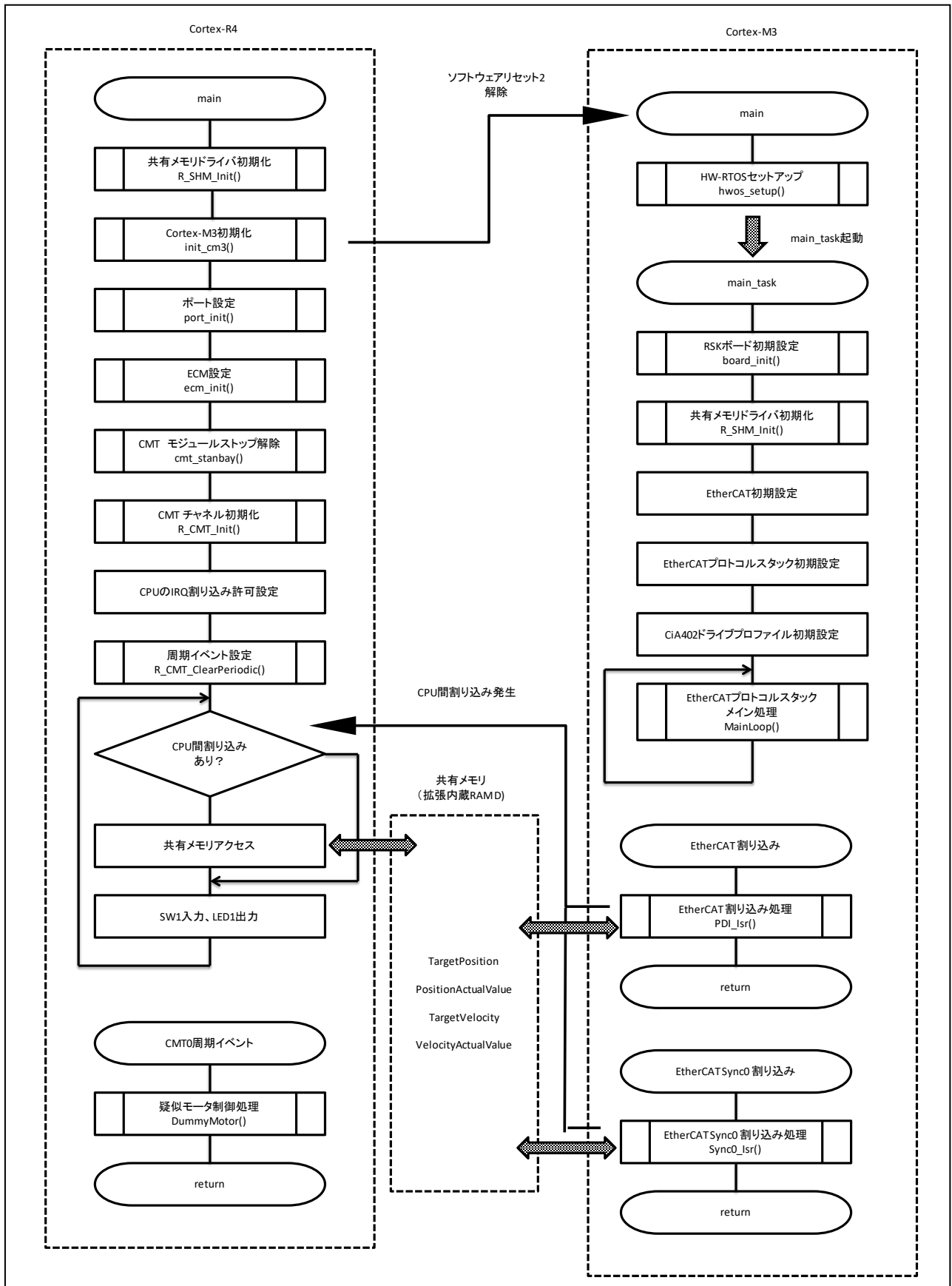
図 5.4 CiA402 サンプル概略フローチャート
