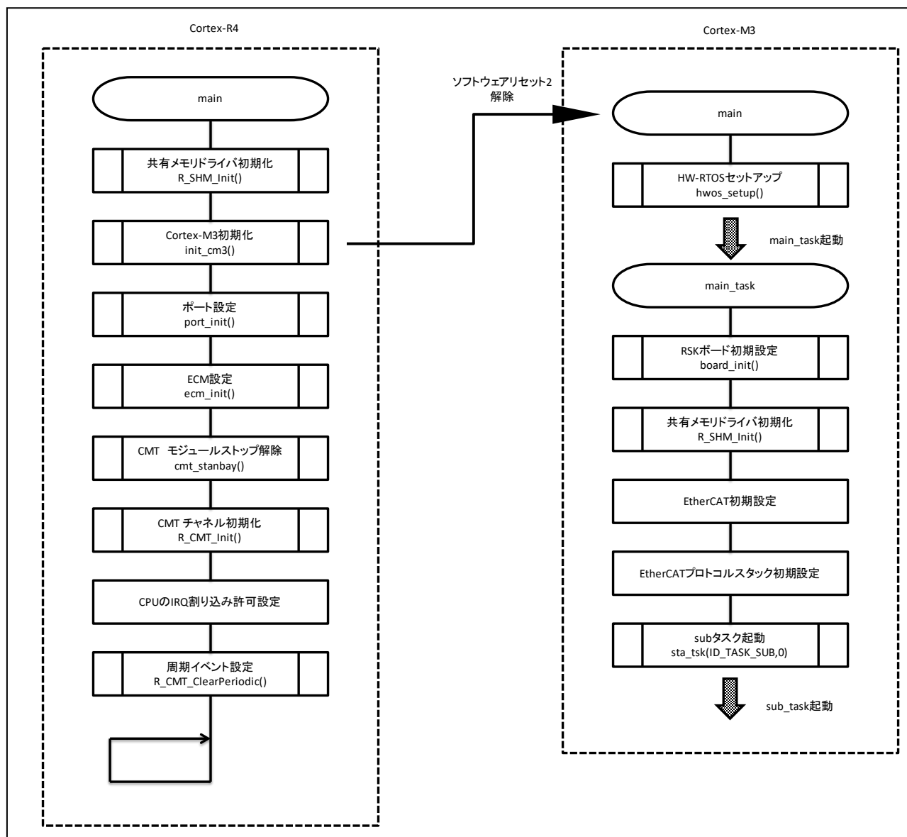
図 5.2 I/O コントローラ・サンプル概略フローチャート 1
