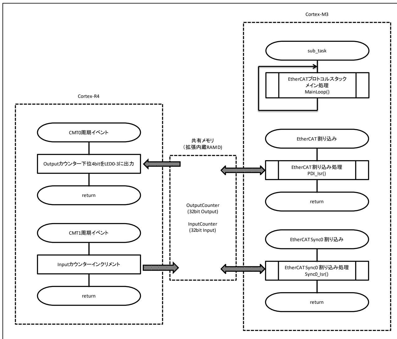
図 5.3 I/O コントローラ・サンプル概略フローチャート 2
