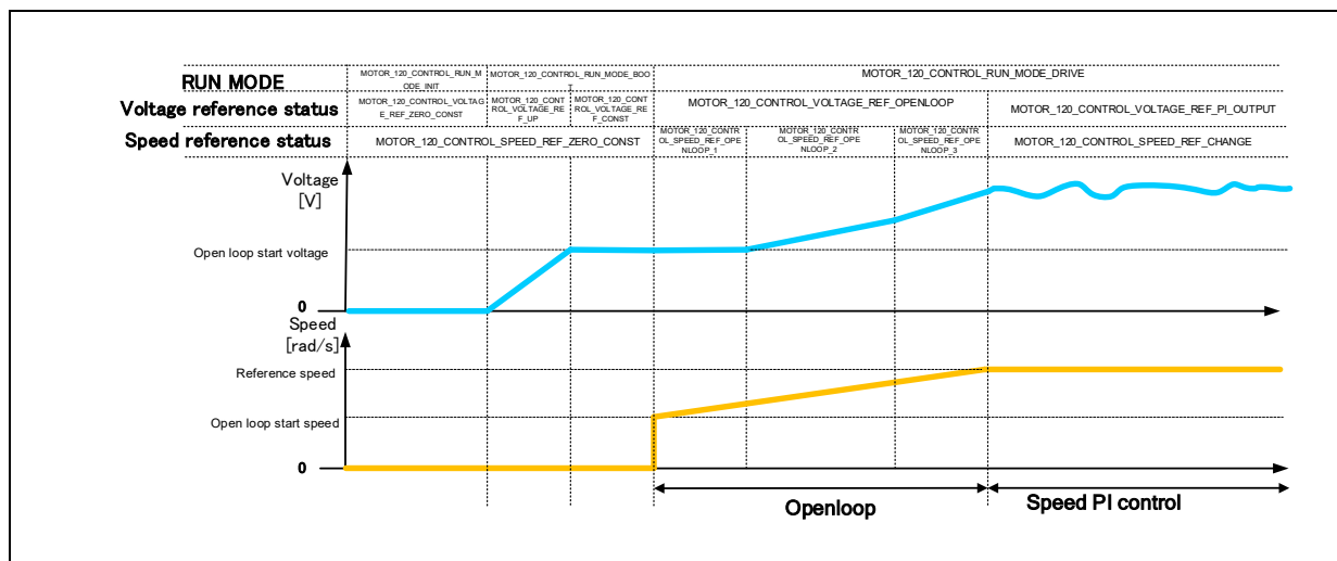
図 3-6 始動方法例
