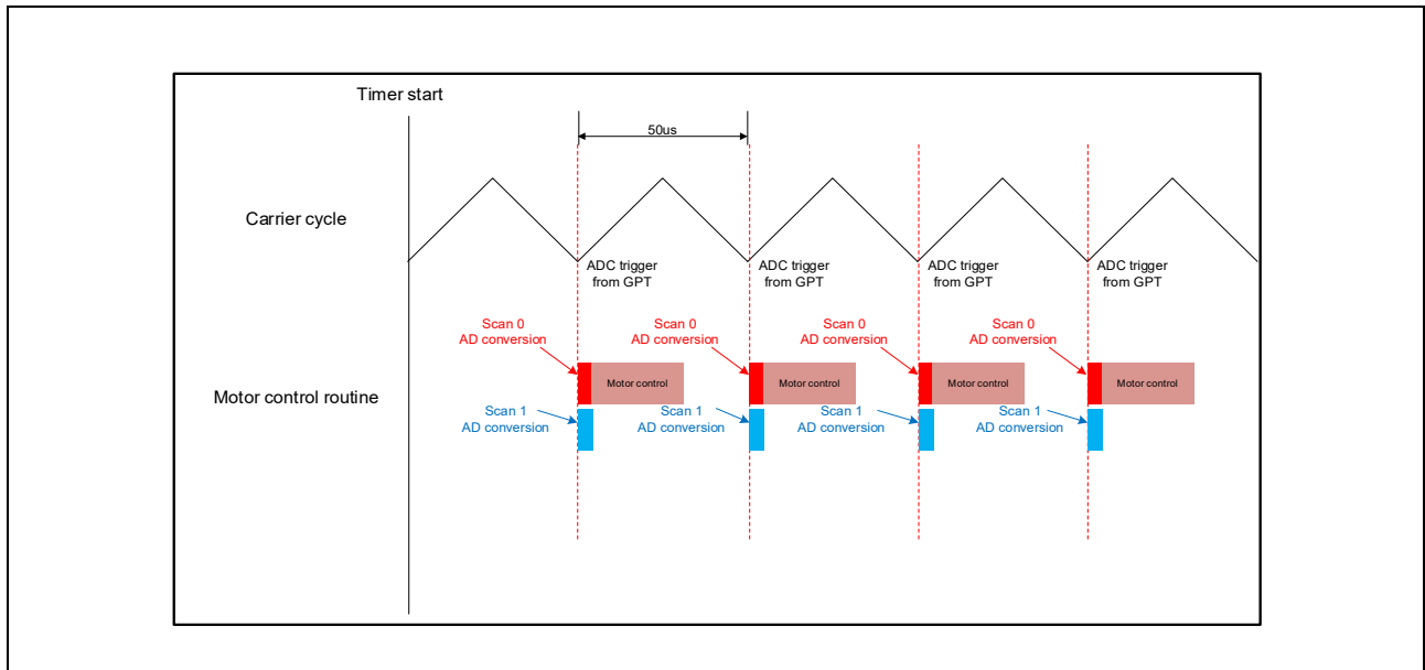
図 3-7 AD トリガタイミング
