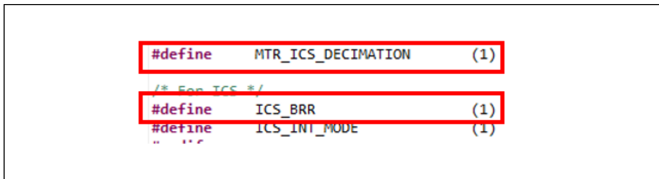
図 4-12 r_mtr_ics.h の修正
