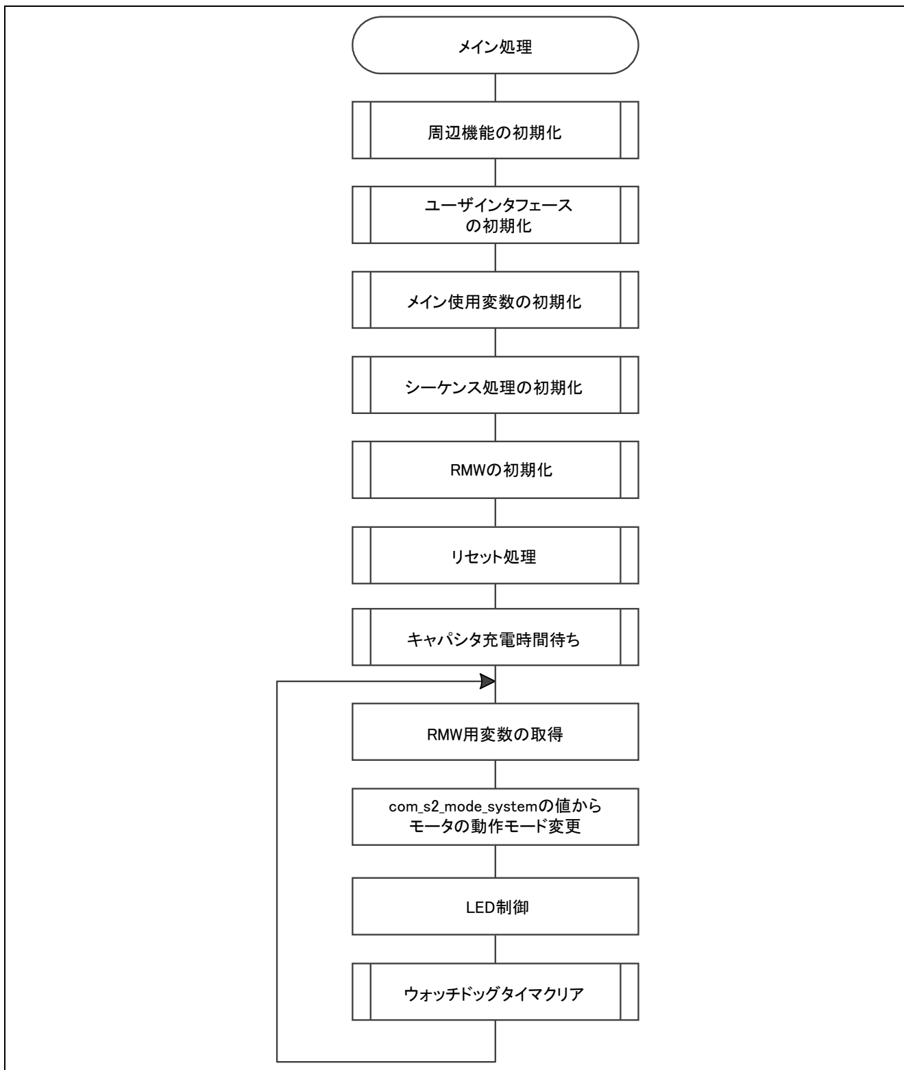
図 3-4 メイン処理
