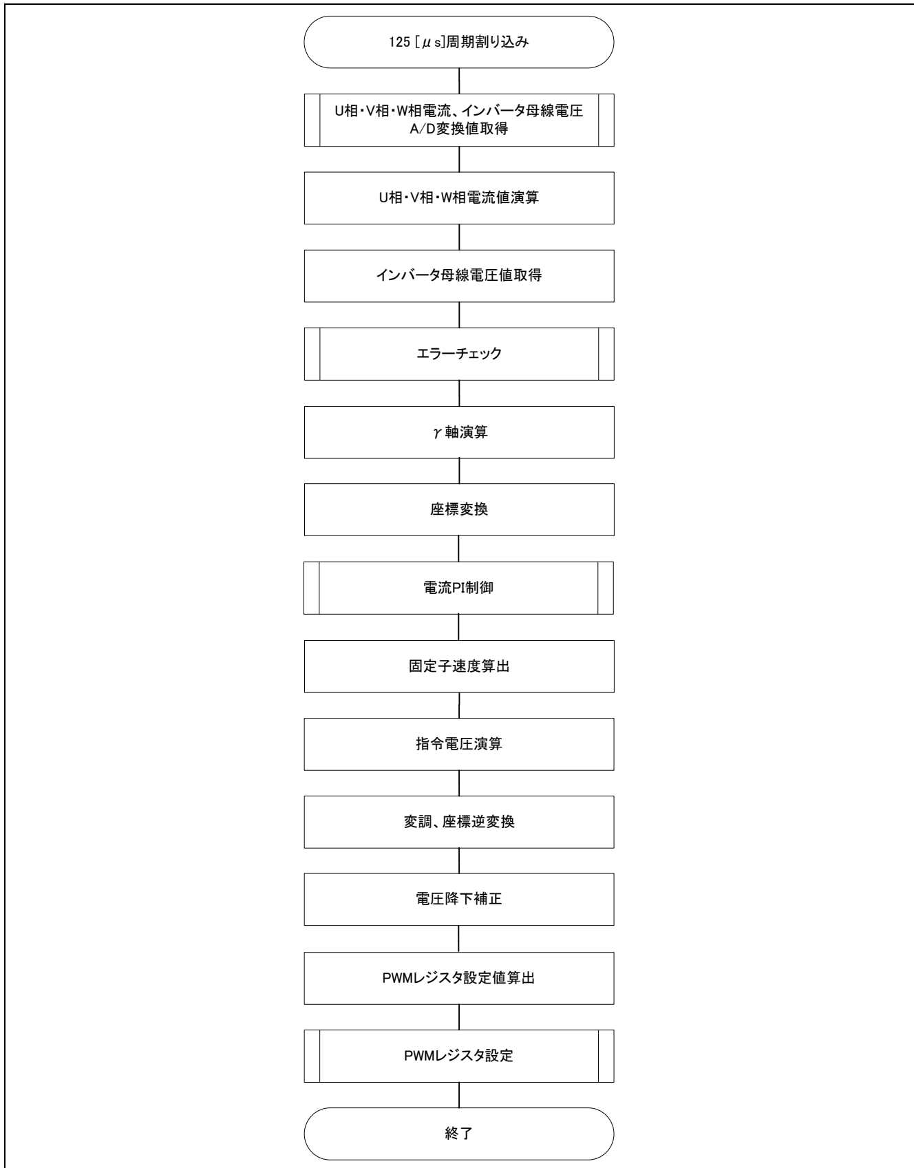
図 3-5 125 [μs]周期割り込み処理
