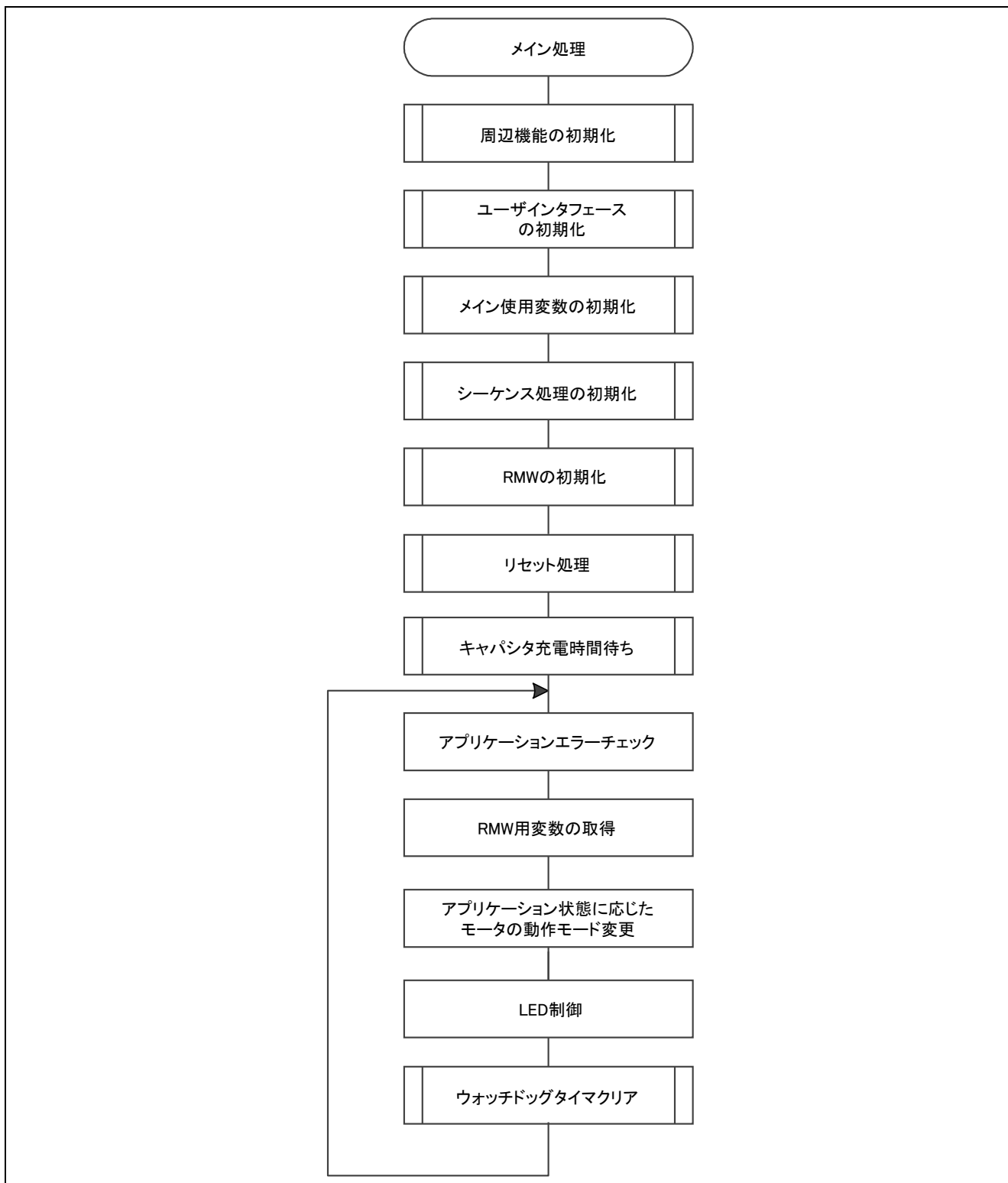
図 3-5 メイン処理
