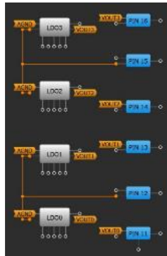
SLG46580の回路例
