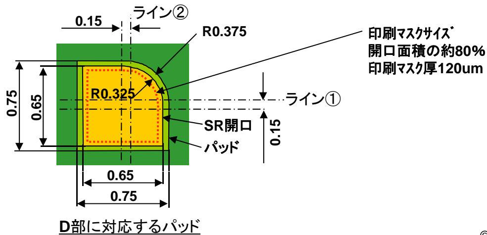
パッケージ側 (Top View)
