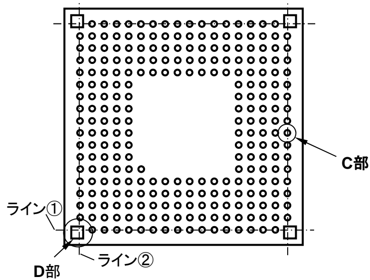
パッケージ側 (Top View)
