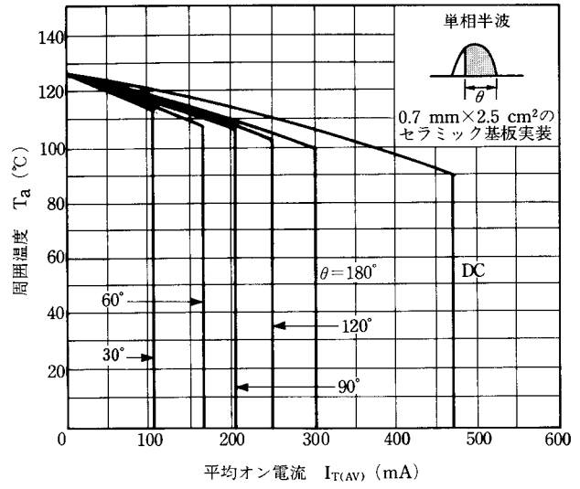
図10 I_{T(AV)}-T_a 定格
