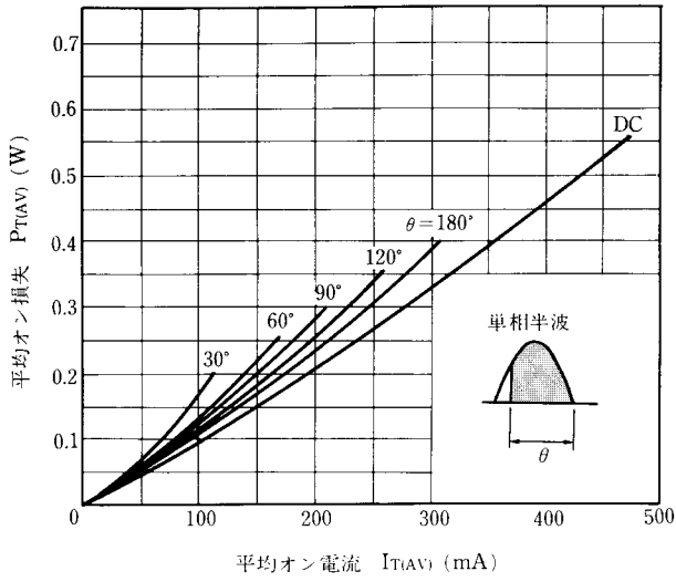
図9 P_{T(AV)}-I_{T(AV)} 特性
