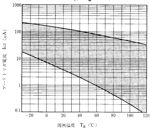
図5 I_{GT}-T_a 特性例
