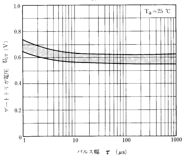
図8 v_{GT}-\tau 特性例
