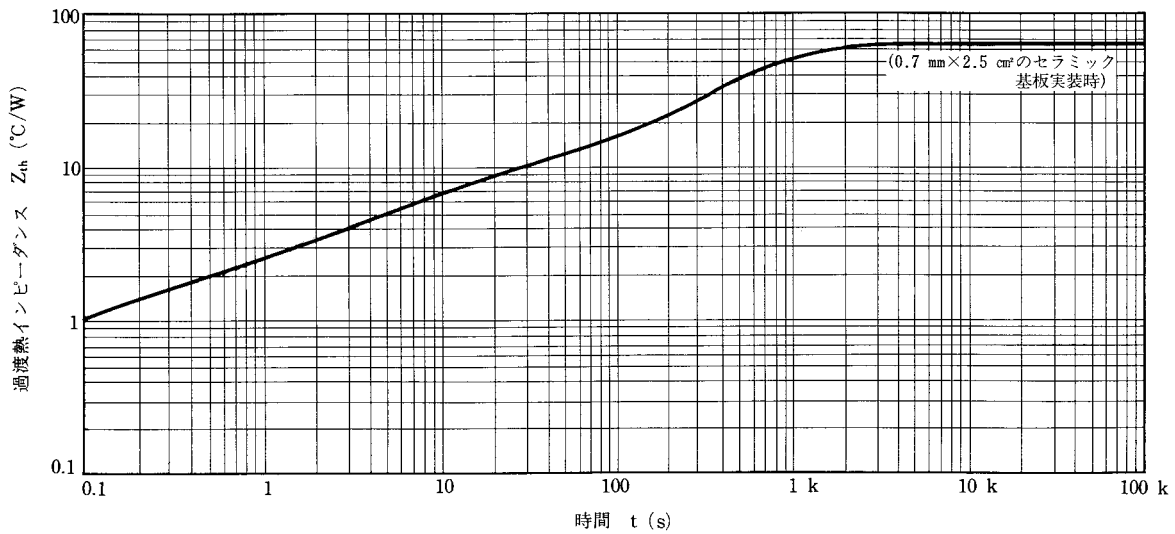
図13 Z_{th} 特性
