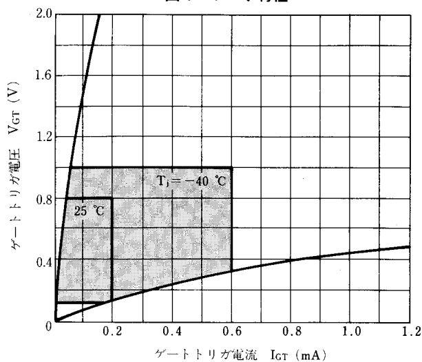
図4 ゲート特性
