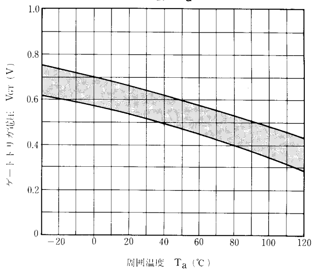
図6 V_{GT}-T_a 特性例
