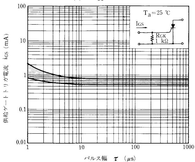
図7 i_{GS}-\tau 特性例
