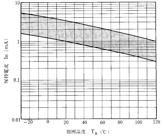
図12 I_H-T_a 特性例
