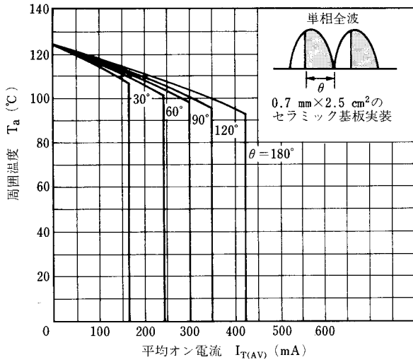
図11 T_a-I_{T(AV)} 定格
