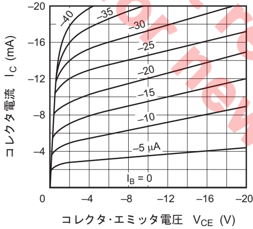
エミッタ接地出力静特性 (2)
