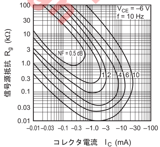
雑音特性 (3)
