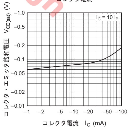
コレクタ・エミッタ飽和電圧対コレクタ電流
