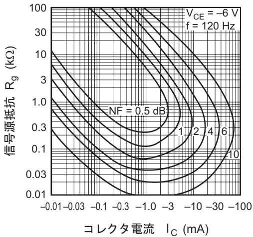
雑音特性 (2)
