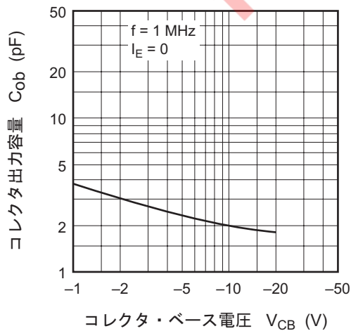
コレクタ出力容量対 コレクタ・ベース電圧
