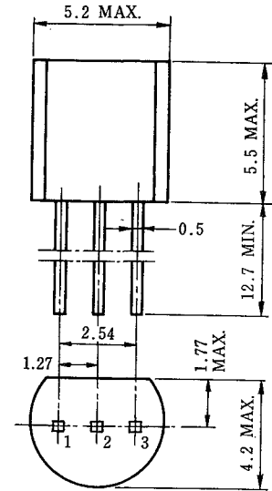
電極接続
