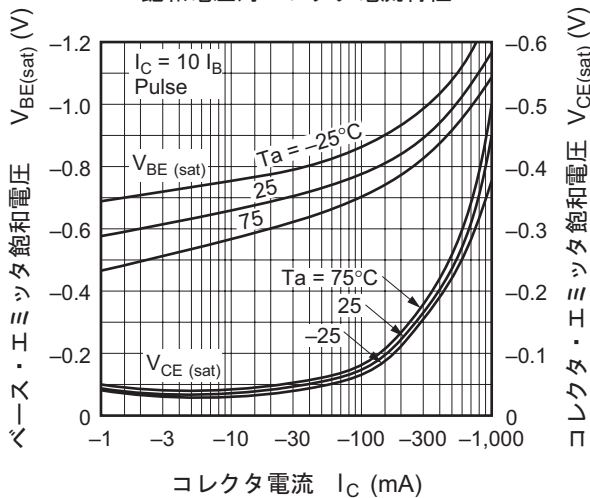
飽和電圧対コレクタ電流特性
