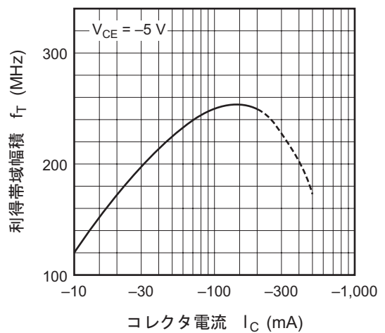
利得帯域幅積対コレクタ電流特性
