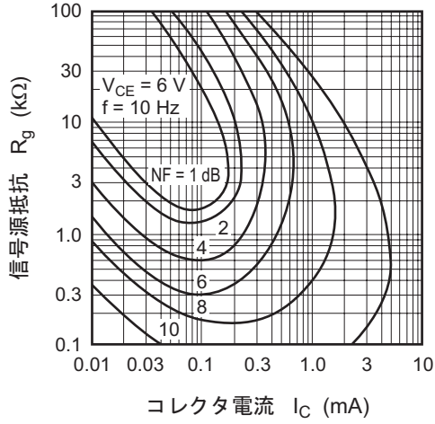
雑音特性
