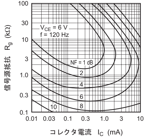
雑音特性
