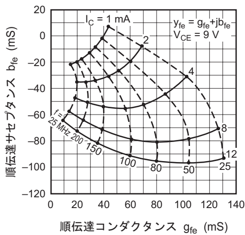
順伝達アドミタンス対周波数特性
