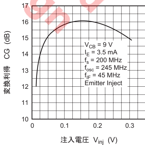
変換利得対注入電圧特性
