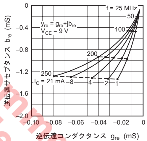
逆伝達アドミタンス対周波数特性
