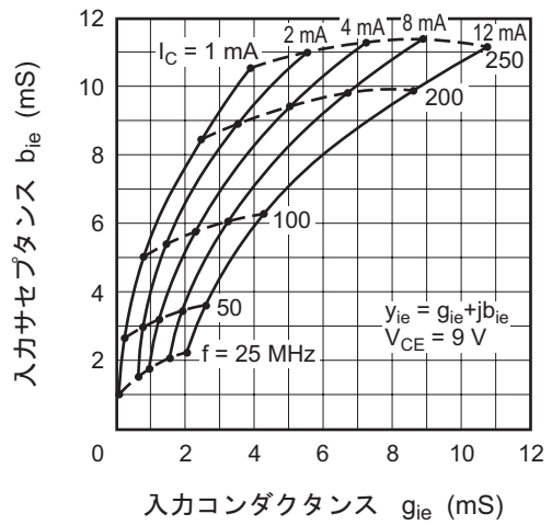
入力アドミタンス対周波数特性
