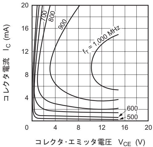
利得帯域幅積曲線
