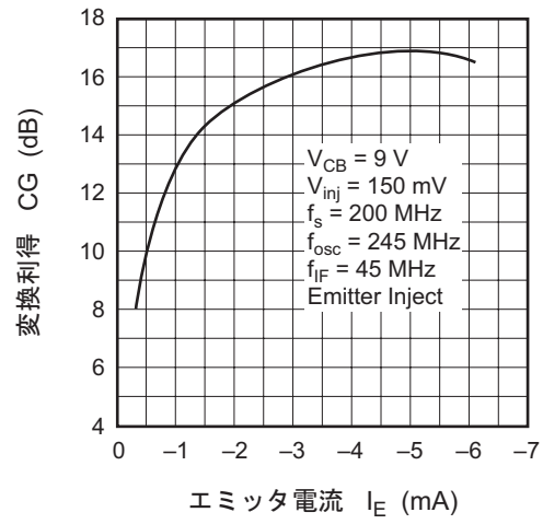
変換利得対エミッタ電流
