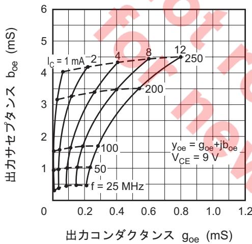
出カアドミタンス対周波数特性
