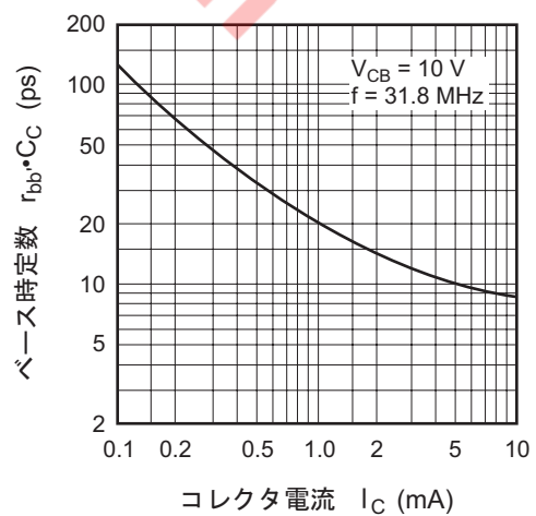
ベース時定数対コレクタ電流特性
