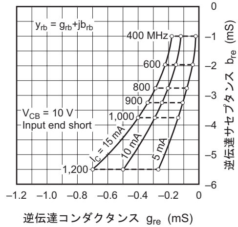
逆伝達アドミタンス特性
