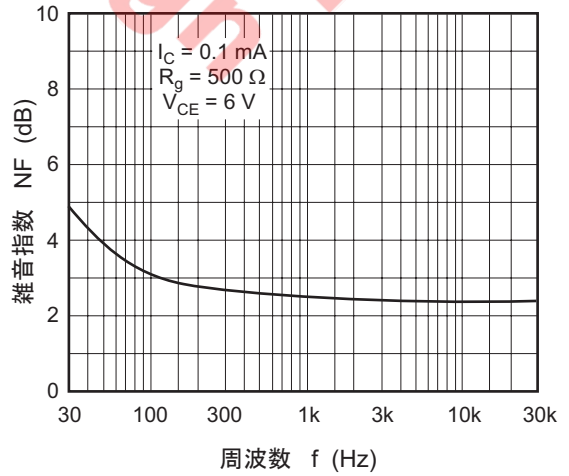
雑音指数対周波数特性
