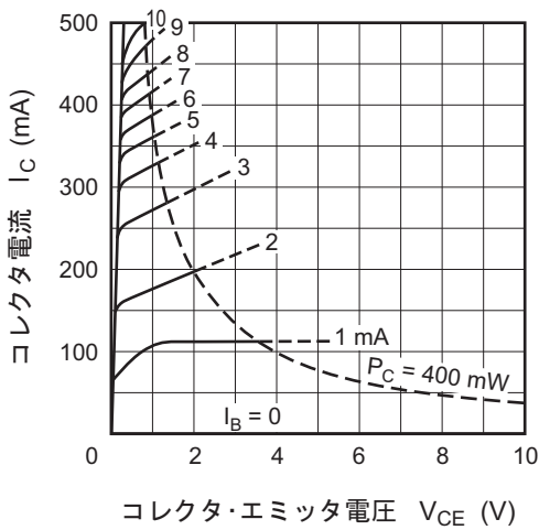
エミッタ接地出力静特性 (2)
