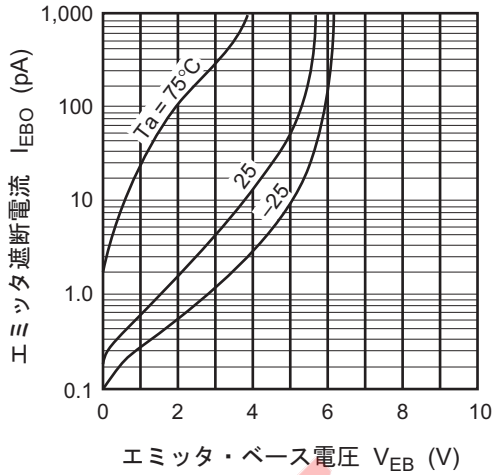
エミッタ遮断電流対 エミッタ・ベース電圧特性
