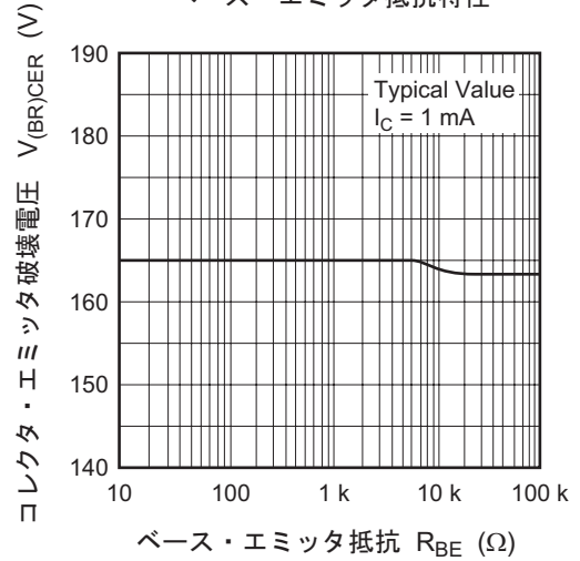
コレクタ・エミッタ破壊電圧対 ベース・エミッタ抵抗特性
