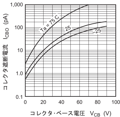
コレクタ遮断電流対コレクタ・ベース電圧特性
