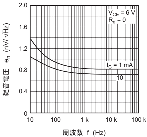
雑音電圧対周波数特性
