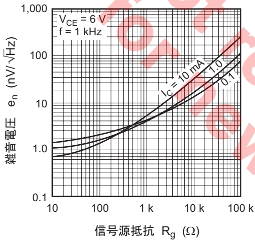
雑音電圧対信号源抵抗特性
