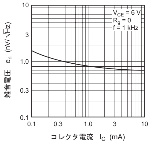
雑音電圧対コレクタ電流特性
