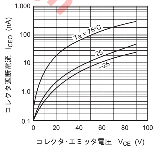
コレクタ遮断電流対コレクタ・エミッタ電圧特性
