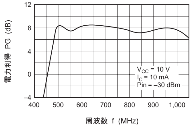
電力利得対周波数特性
