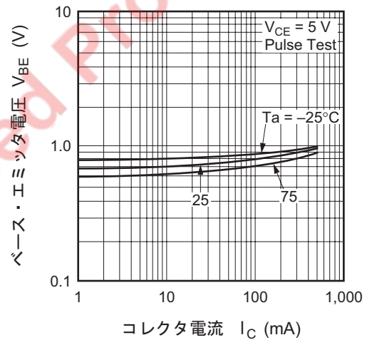
ベース・エミッタ電圧対コレクタ電流特性
