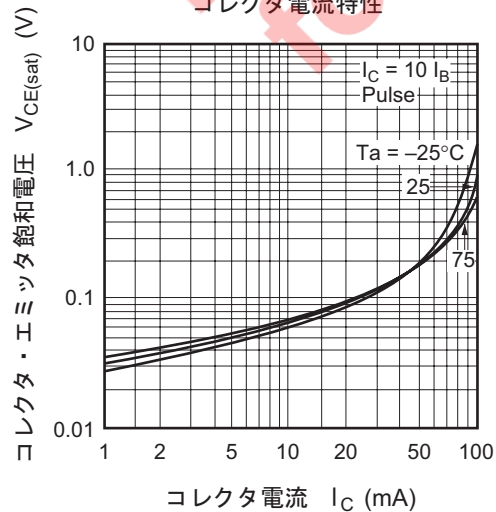
コレクタ・エミッタ飽和電圧対コレクタ電流特性
