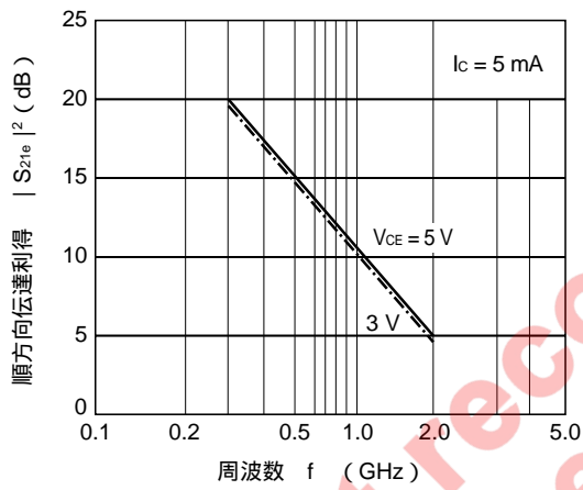
|S_{21e}|^2 - f 特性
