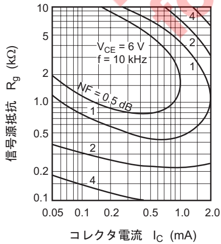
雑音特性
