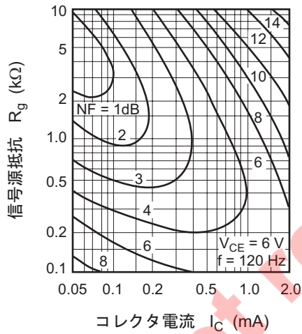
雑音特性
