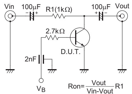
オン抵抗測定回路
