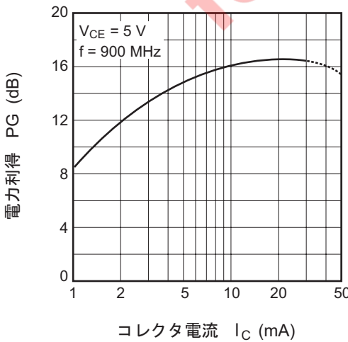
電力利得対コレクタ電流特性
