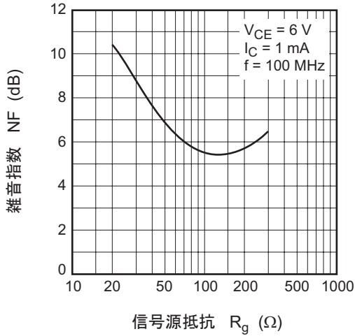
雑音指数対信号源抵抗特性
