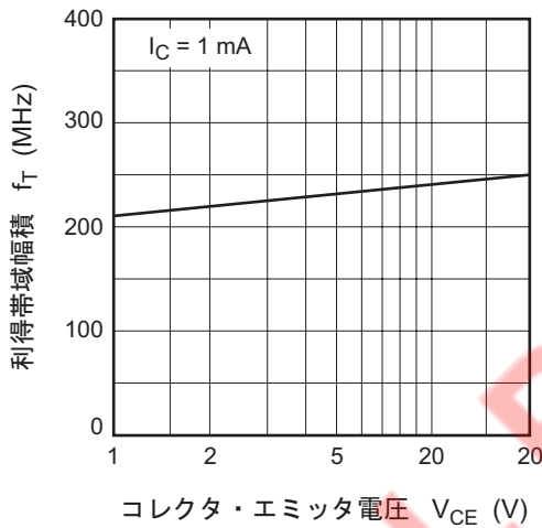
利得帯域幅積対コレクタ・エミッタ電圧
