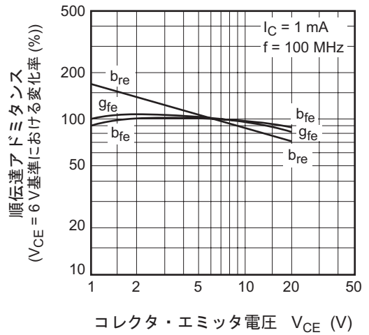
順伝達アドミタンス対コレクタ・エミッタ電圧特性
