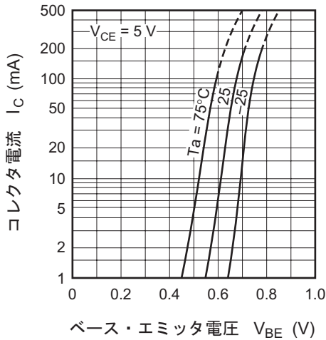
エミッタ接地伝達静特性
