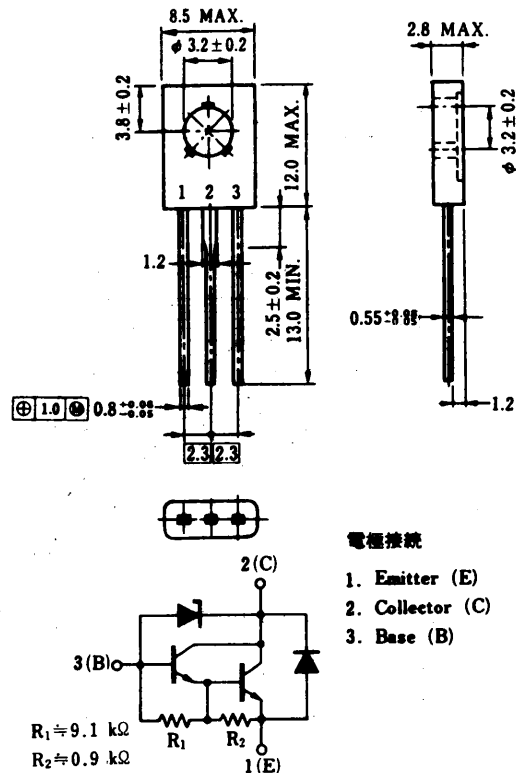
外形図(単位: mm)
