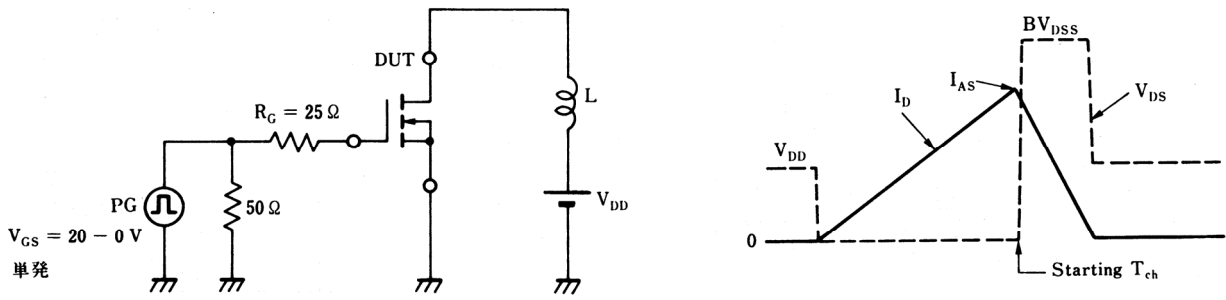
測定回路図 1：アバランシェ耐量測定回路
