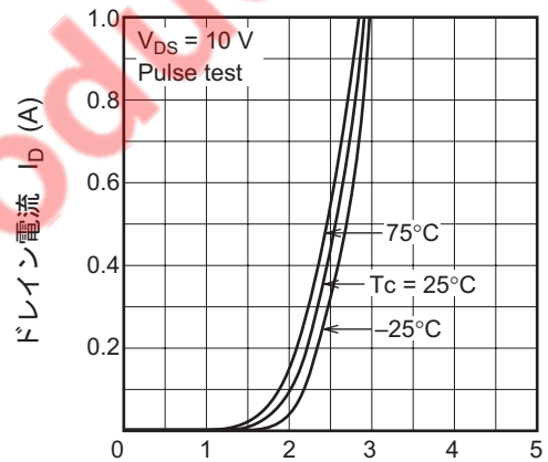
ソース接地伝達静特性
