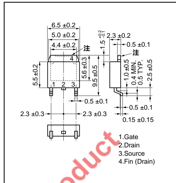
2)TO-252 (MP-3Z)
