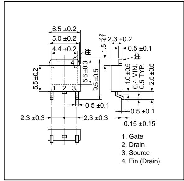
★ 2) TO-252 (MP-3Z)
