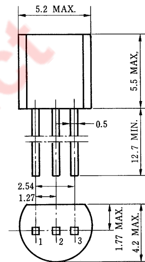
外形図 (Unit: mm)
