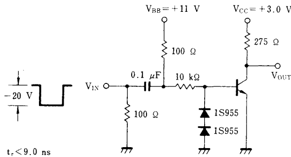
t_{off} 測定回路
