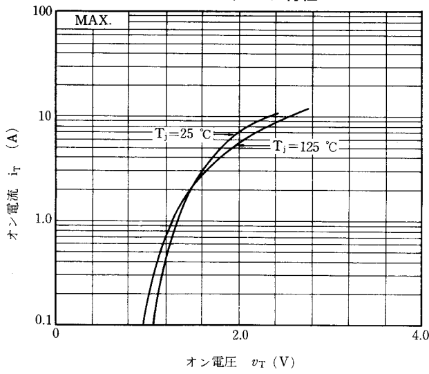
図1 i_T-v_T 特性
