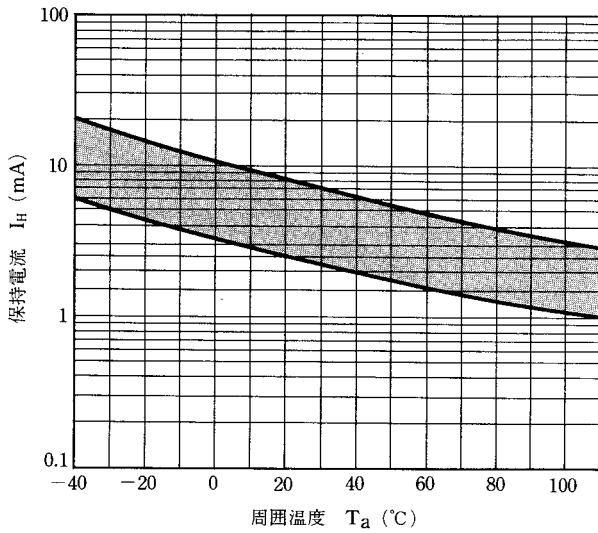
図9 I_H-T_a 特性例
