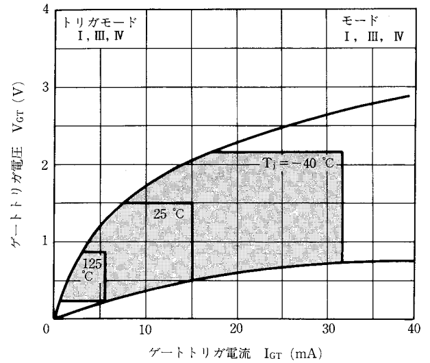
図4 V_{GT}-I_{GT} 特性例
