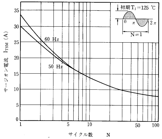
図2 I_{TSM} 定格
