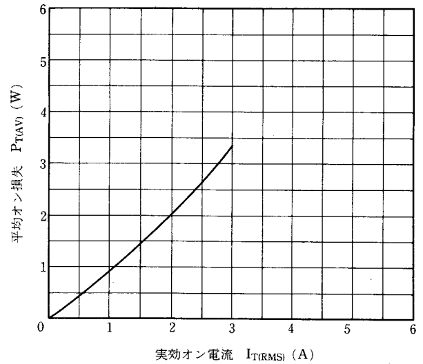
図10 P_{T(AV)}-I_{T(RMS)} 特性
