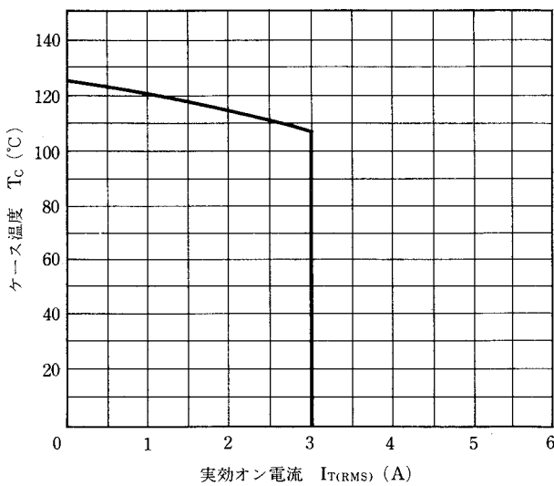
図11 T_C-I_{T(RMS)} 定格
