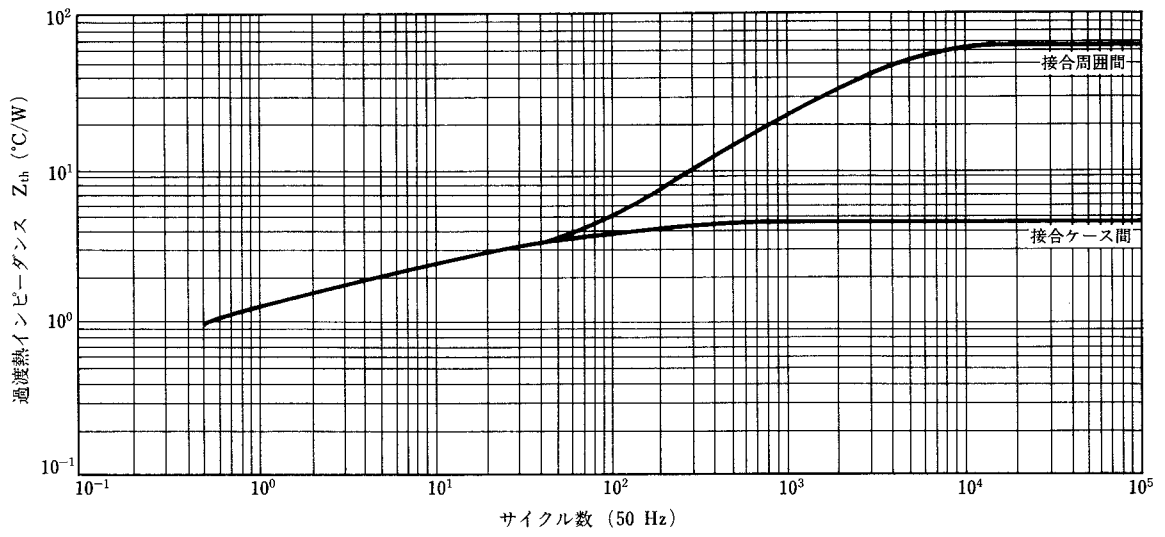
図13 Z_{th} 特性
