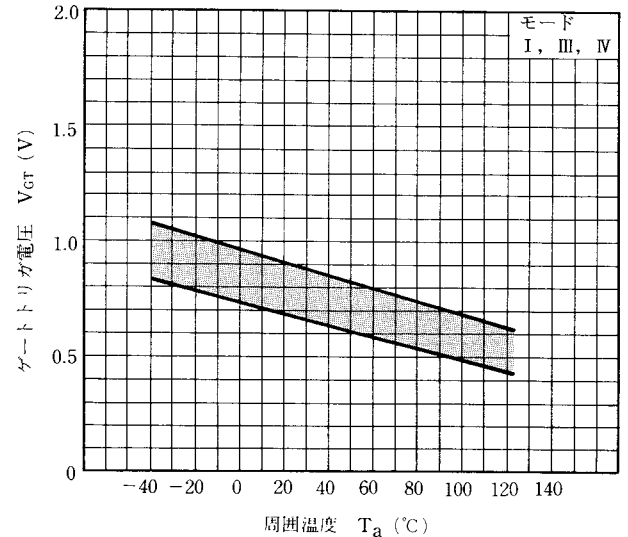
図6 V_{GT}-T_a 特性例
