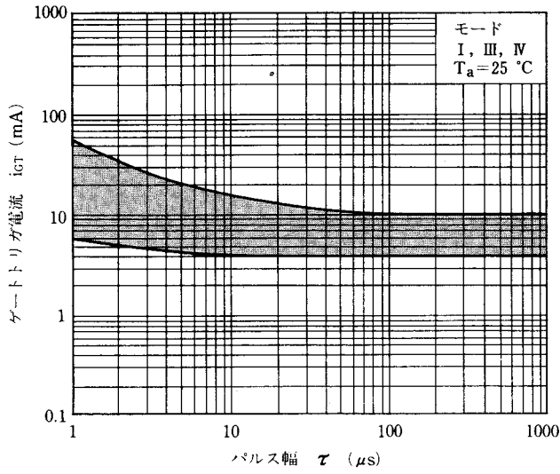
図7 i_{GT}-\tau 特性例
